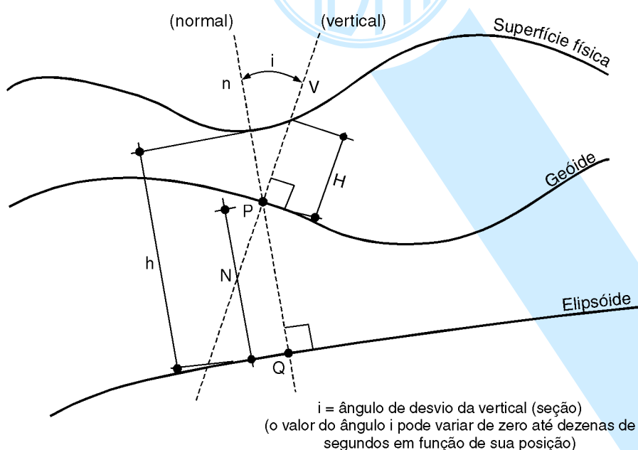
Figura 1 - Esquema dos conceitos de vertical, normal e altura
