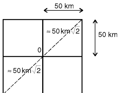
Figura 3 - Origem do Sistema Topográfico Local e distância máxima a esta origem
