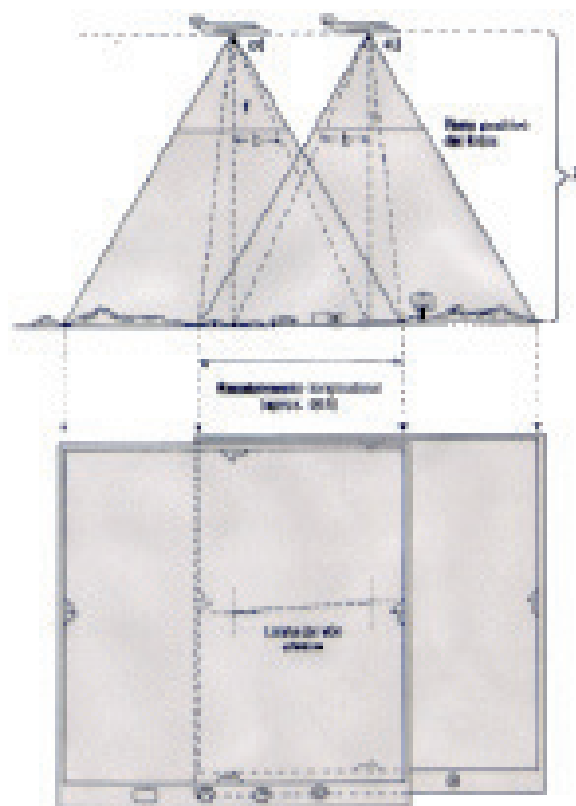
Figura 4.3 - Recobrimento Longitudinal
