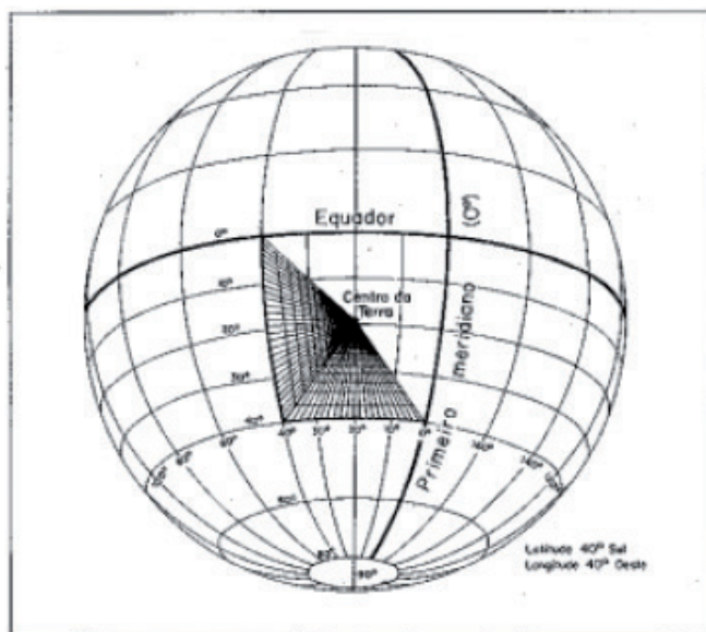
Figura 2.3 - Latitude e Longitude
