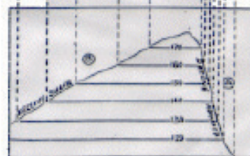
Figura 3.13 - Formação escarpada e suave
