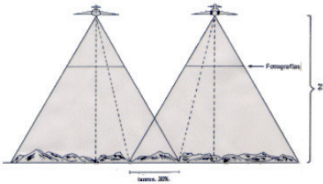
Figura 4.4 - Recobrimento lateral
