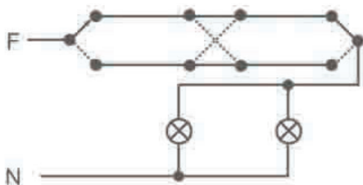
Fig. – Diagrama multifilar de interruptores intermediários ( four-way ) com quatro comandos
