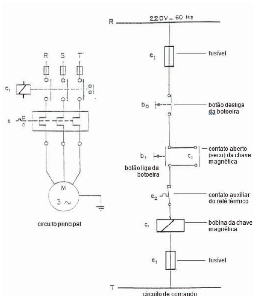
Fig. – Diagrama com destaque para circuito principal e circuito de comando
