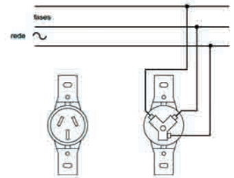
Fig. – Tomada 3p
