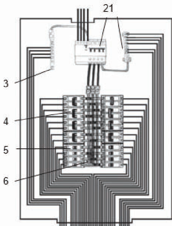
Fig. – QD para fornecimento trifásico
