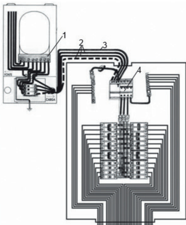
Fig. – Circuito de distribuição bifásico ou trifásico protegido por disjuntor termomagnético
