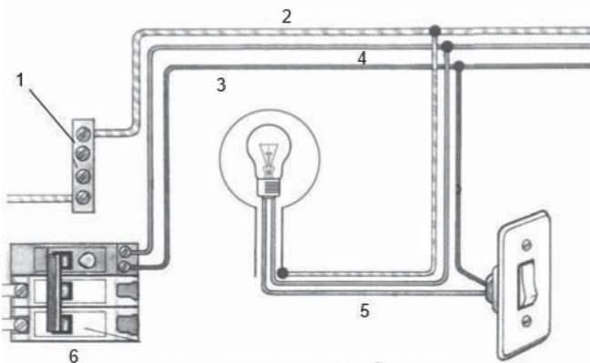
Fig. – Circuito de iluminação externa
