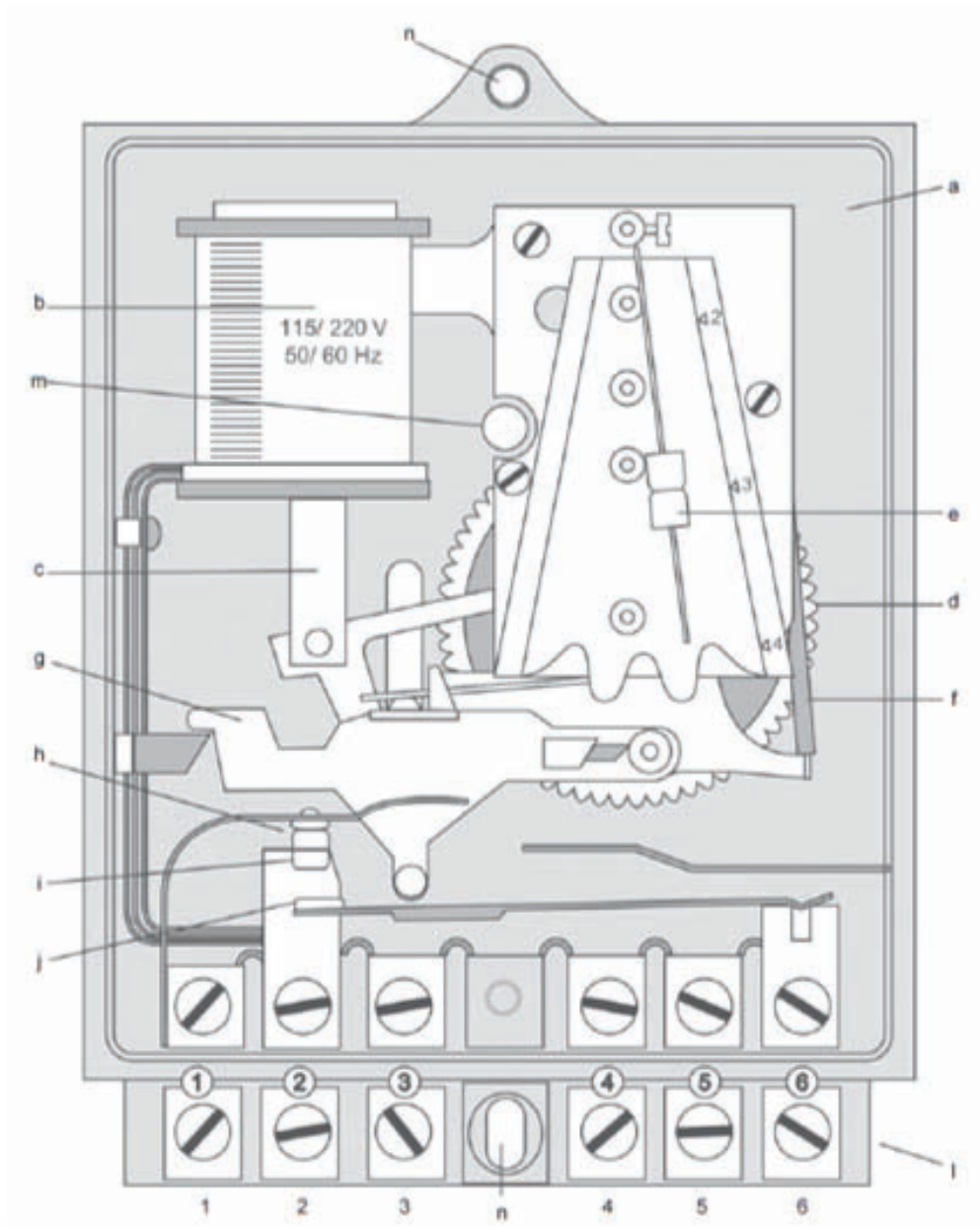
Fig. – Minuteria eletromecânica
