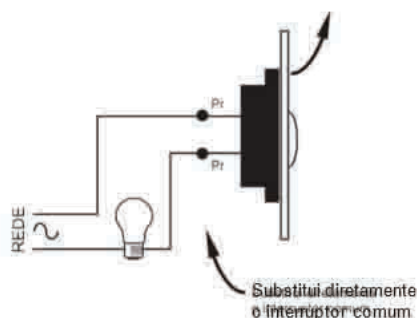
Fig. – Ligação de sensor com 2 fios
