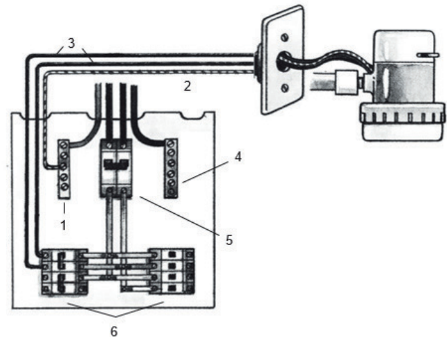
Fig. – Circuito de tomada de uso específico (220V)
