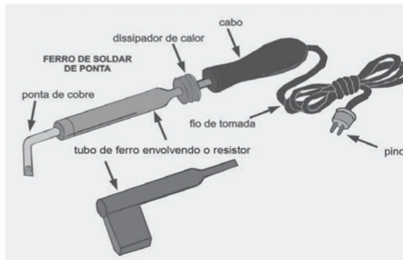
Fig. – Ferro de soldar e seus componentes
