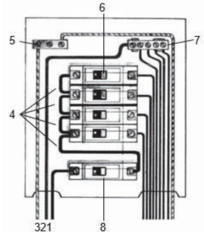
Fig.– QD para fornecimento monofásico
