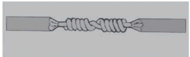
Fig. – Emenda em prosseguimento
