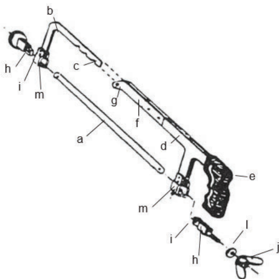
Fig. – Serra manual e seus elementos
