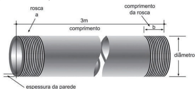
Fig. – Elementos do eletroduto
