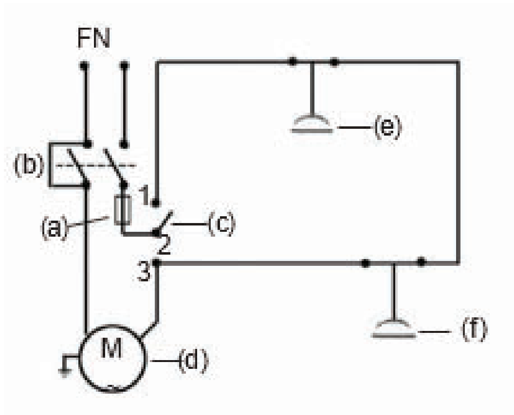
Fig. – Diagrama multifilar de motobomba
