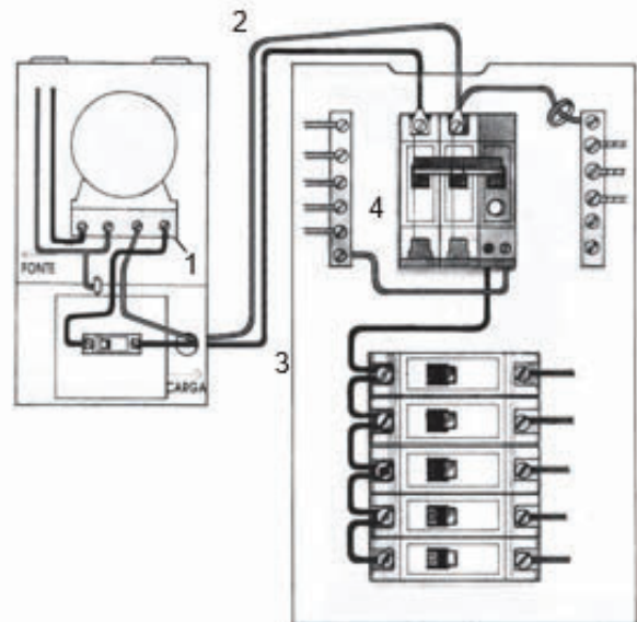
Fig. – Circuito de distribuição monofásico protegido por disjuntor termomagnético
