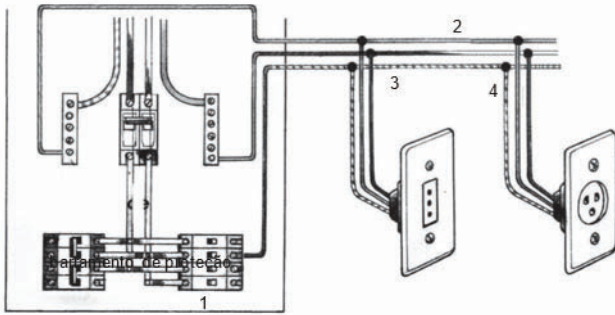
Fig. – Circuito de tomadas de uso geral
