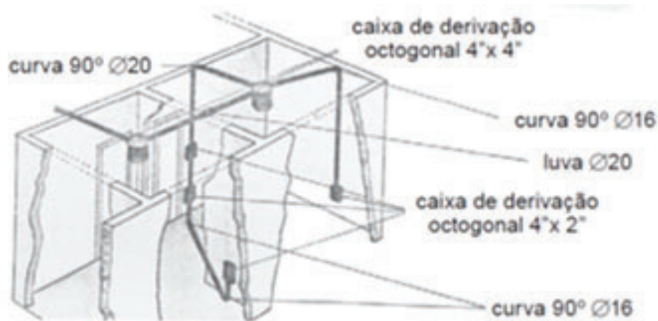
Fig. – Caixas de passagem instaladas
