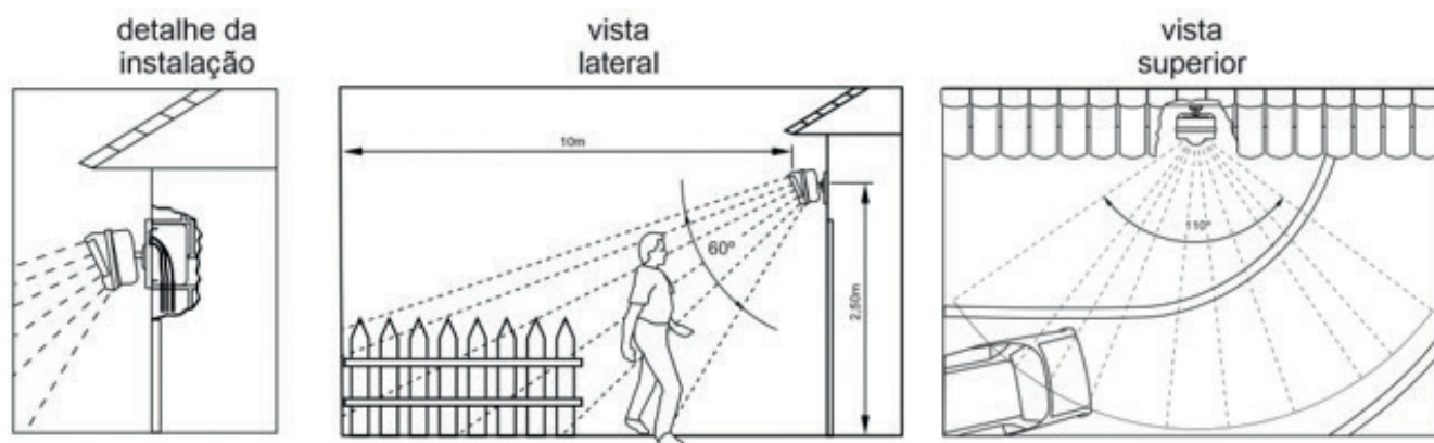
Fig. – Instalação e posicionamento do interruptor automático por presença
