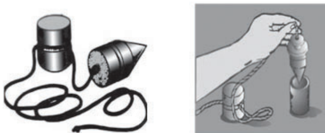
Fig. – Prumo de centro
