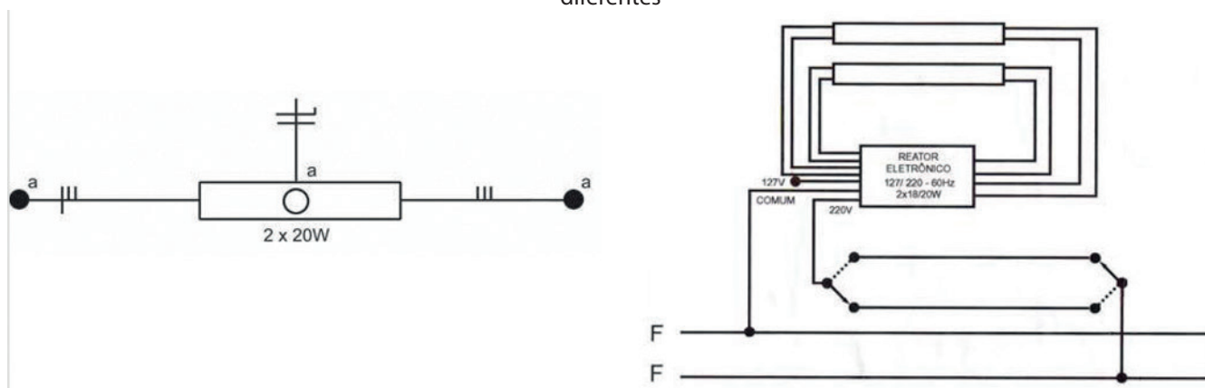
Fig. – Diagrama D3 – Partida rápida eletrônica: duas lâmpadas fluorescentes de 20W – 220V, comandadas de dois pontos diferentes
