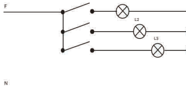
Fig. – Diagrama multifilar com interruptor de três seções unifilar:
