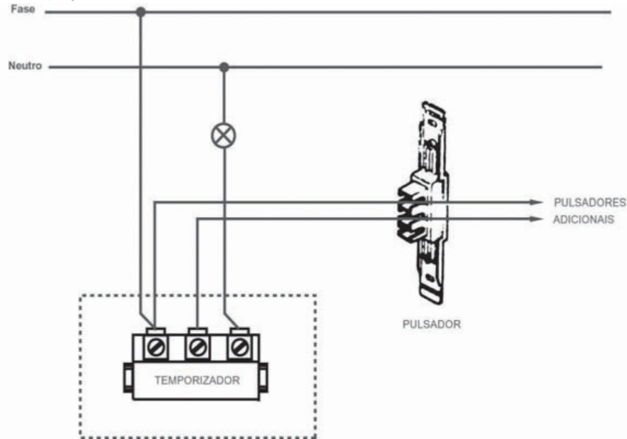
Fig. – Esquema de ligação da minuteria individual
