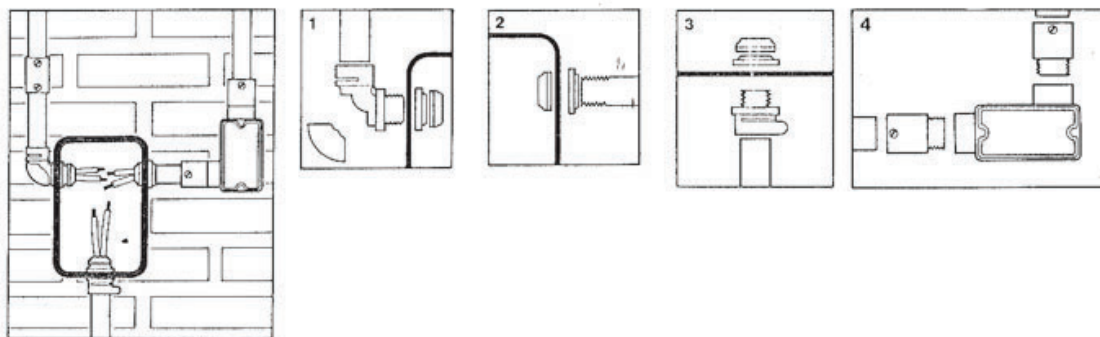
Fig. – Uso de condulete sem rosca
