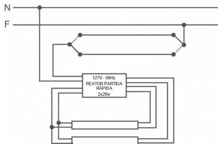
Fig. – Diagrama D2 – Partida rápida eletromagnética: duas lâmpadas fluorescentes de 20W – 127V, comandadas de dois pontos diferentes
