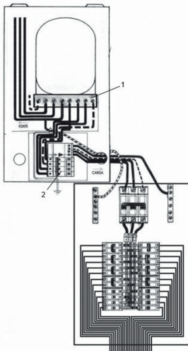
Fig. – Circuito de distribuição bifásico ou trifásico protegido por disjuntor DR
