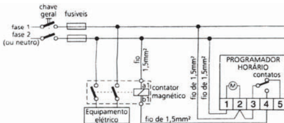
Fig. – Ligação dos fios para fornecimento de energia ao programador horário com equipamentos elétricos monofásicos, que consomem energia acima da capacidade dos contatos de saída
