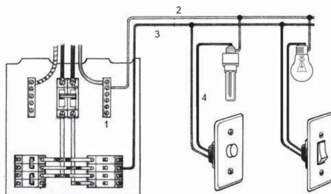
Fig. – Circuito de iluminação para disjuntor monopolar
