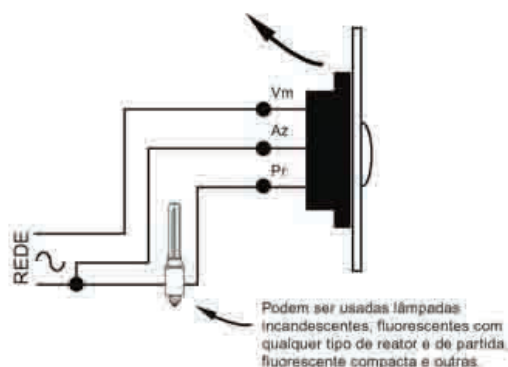
Fig. – Ligação de sensor com 3 fios
