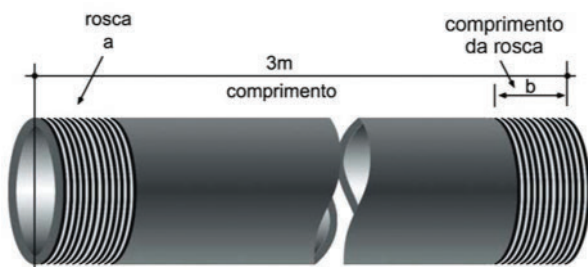
Fig. – Eletroduto rígido metálico
