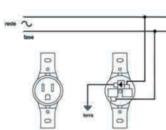
Fig. – Tomada 2p+t
