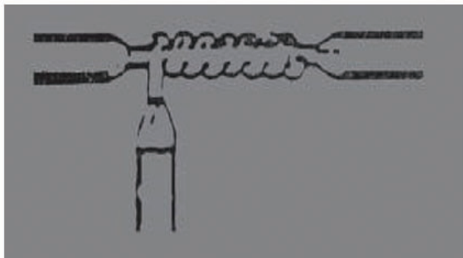
Fig. – Fazendo a emenda
