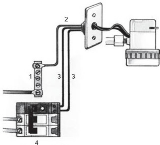
Fig. – Circuito de tomada de uso específico (220V)
