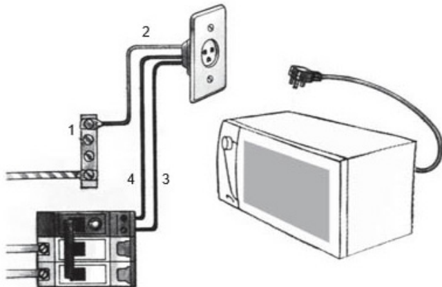
Fig. – Circuito de tomada de uso específico (127V)
