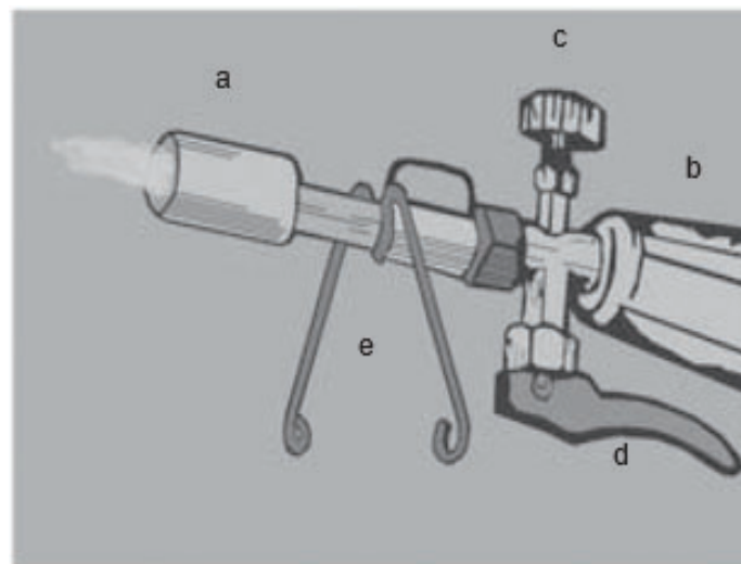
Fig. – Maçarico a gás
