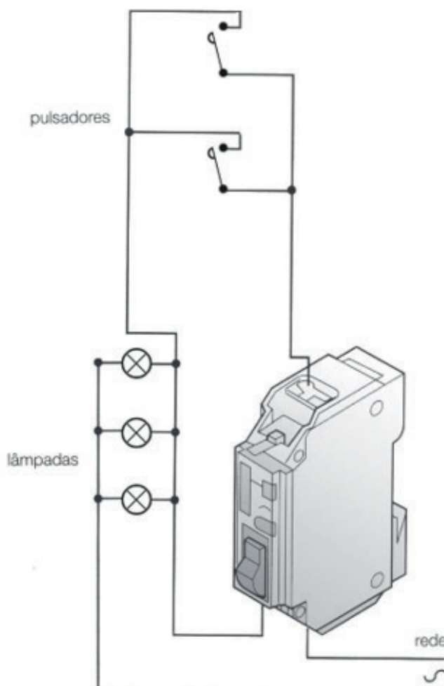
Fig. – Esquema de ligação da minuteria eletrônica
