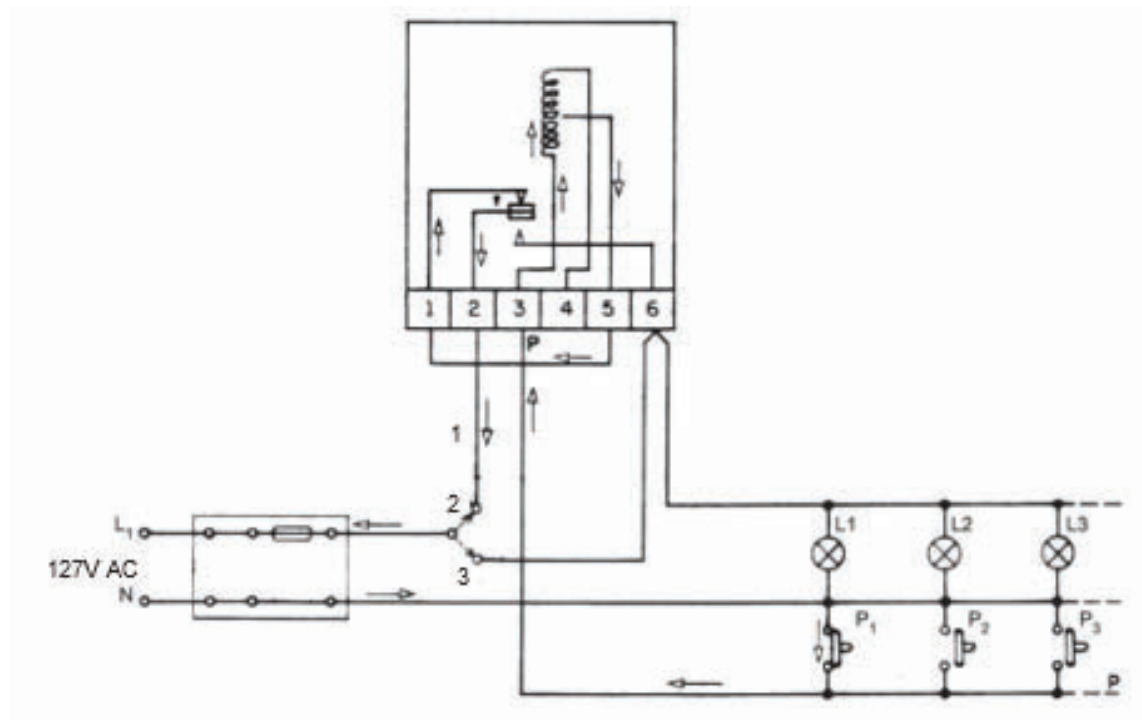
Fig. – Diagrama de circuito de minuteria eletromagnética, chave seletora, lâmpadas e pulsadores
