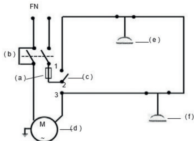
Fig. – Diagrama multifilar de motobomba
