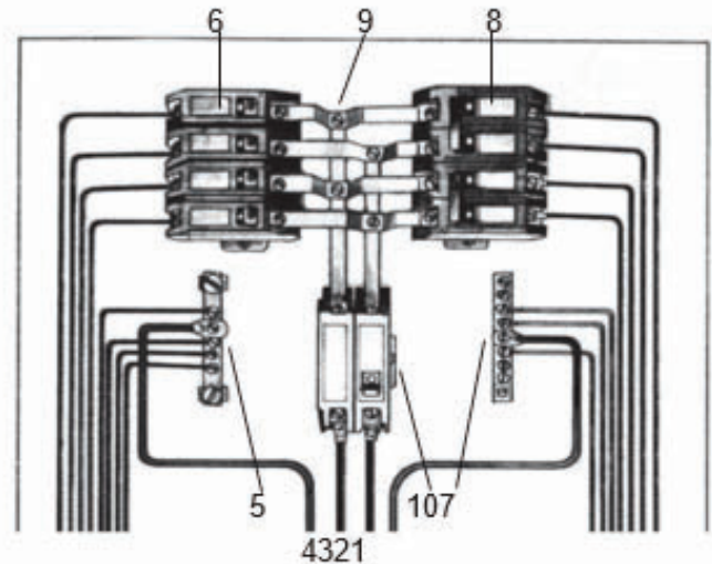
Fig.– QD para fornecimento bifásico
