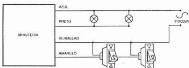
Fig. – Esquema de ligação da minuteria modular universal
