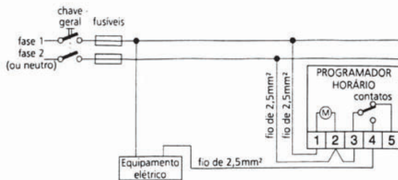
Fig. – Ligação dos fios para fornecimento de energia ao programador horário com equipamentos elétricos monofásicos, que consomem energia dentro da capacidade dos contatos de saída
