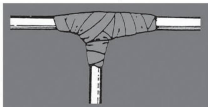
Fig. – Isolando a emenda em derivação
