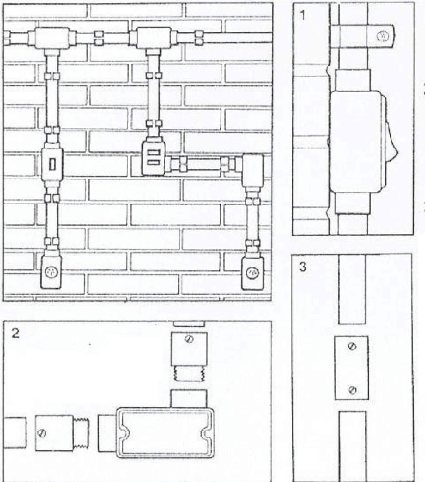
Fig. – Uso de condutes
