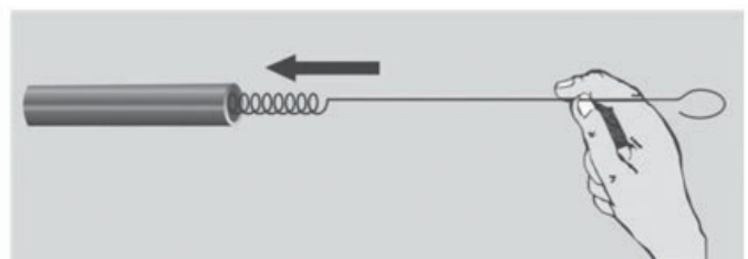
Fig. – Inserindo a mola no eletroduto
