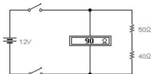
Figura 49: Medição Ohmímetro Digital
