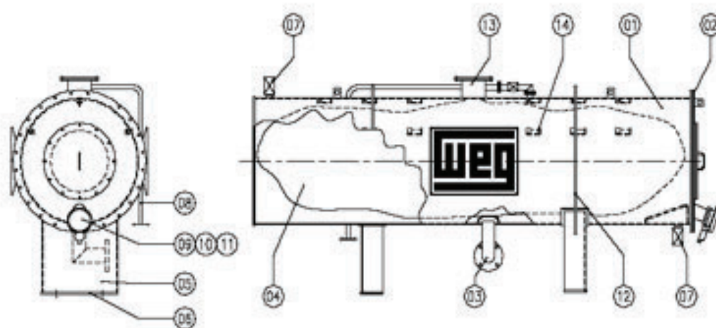
Figura 9 – Conservador de óleo com bolsa de borracha
