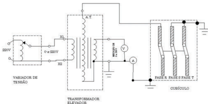
Figura 91: Ensaio de Tensão Aplicada.
