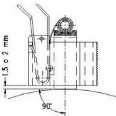
Figura 84: Porta Escovas.
