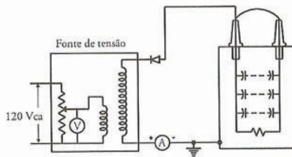
FIGURA – TESTE DE TENSÃO APLICADA VCC ENTRE OS TERMINAIS E A CAIXA
