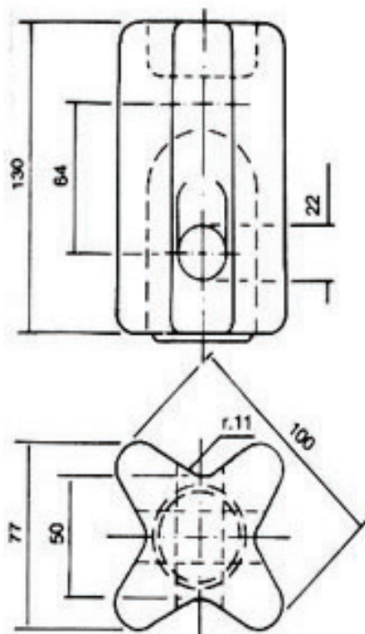
FIGURA 19 - ISOLADOR TIPO CASTANHA
