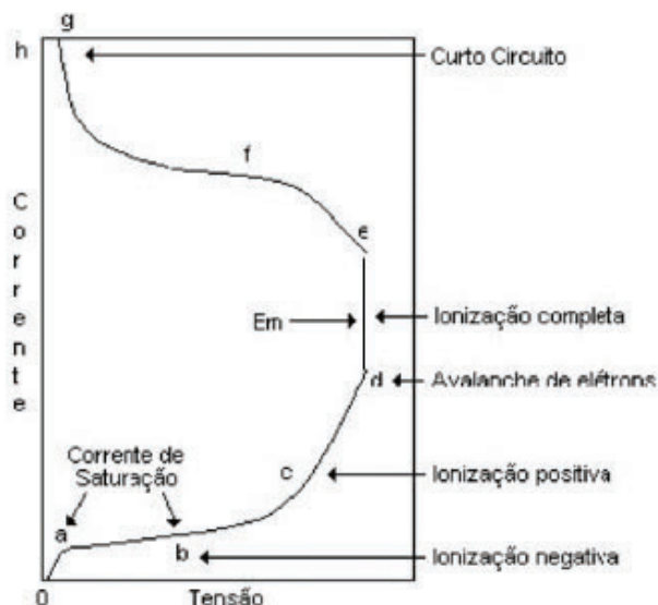
Figura 01- Características de ionização e ruptura nos gases
