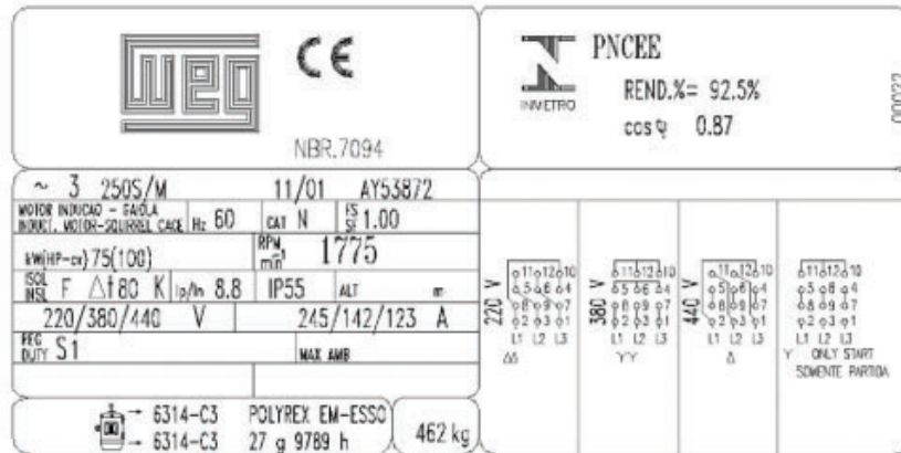
Figura 65: Placa e Identificação de Motor Trifásico
