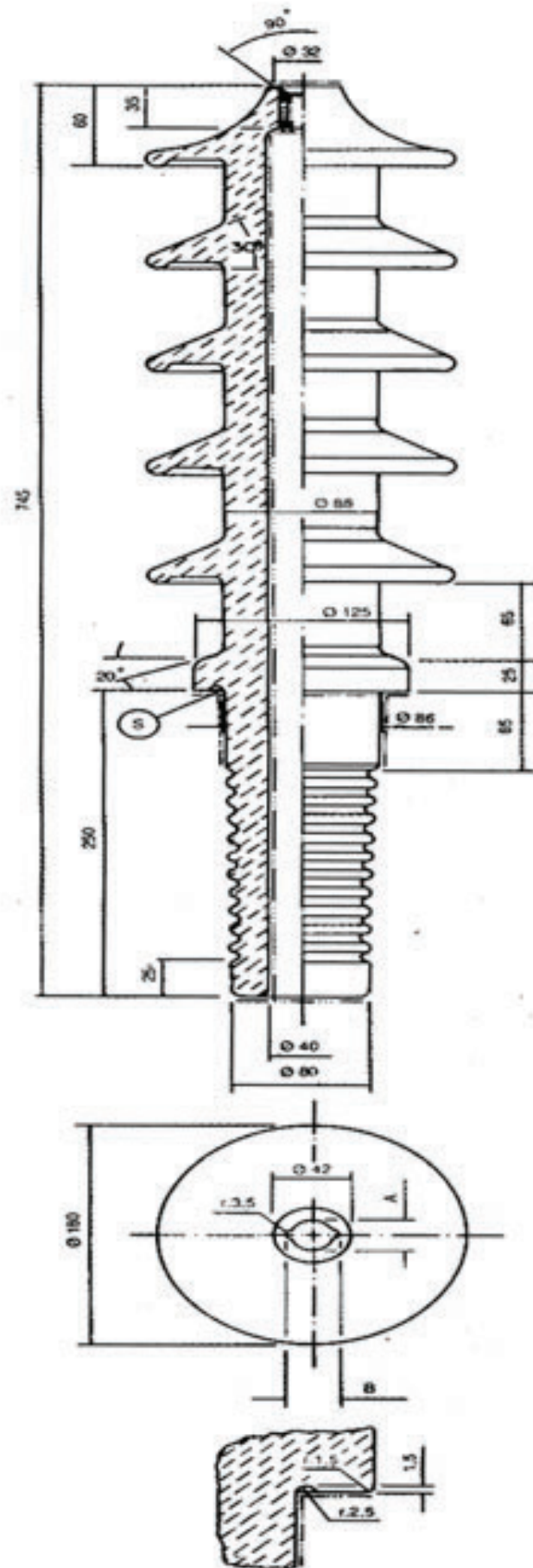
FIGURA 24 - ISOLADOR TIPO BUCHA TRAFO
