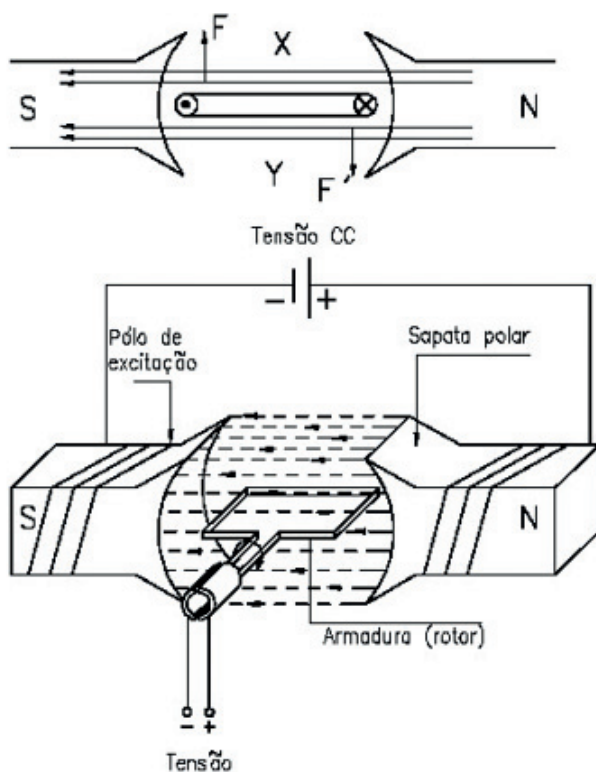
Figura 81: Princípios de funcionamento.
