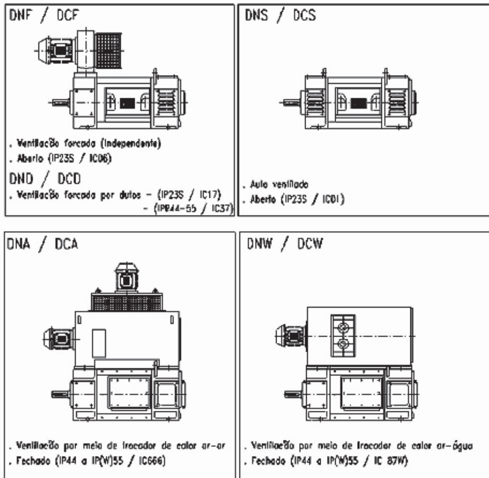
Figura 79: Tipos de ventilação.
