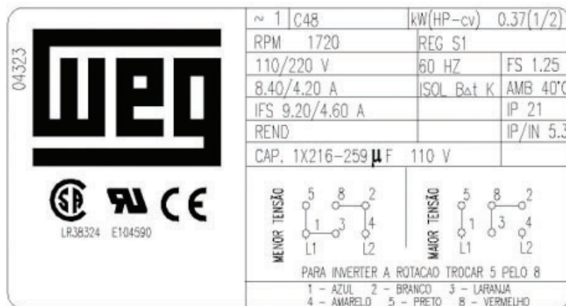
Figura 66: Placa e Identificação de Motor Monofásico
