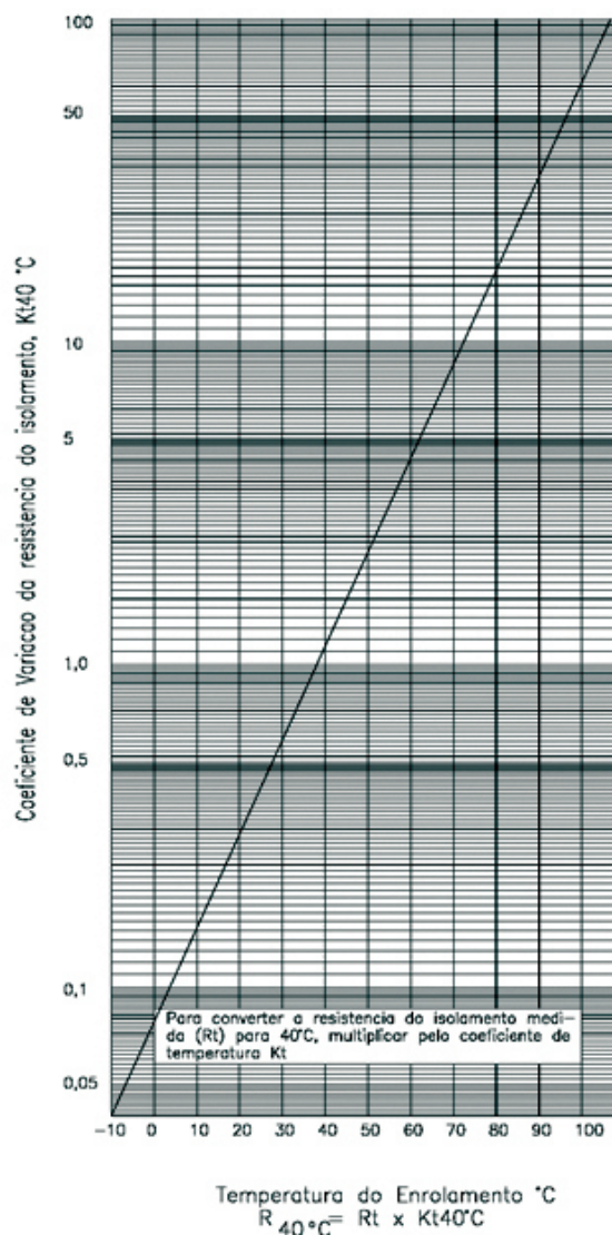
Figura 76: Tabela - Variação da resistência de Isolamento em função da temperatura do enrolamento
