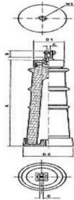
FIGURA 20 - ISOLADOR TIPO SUPORTE
