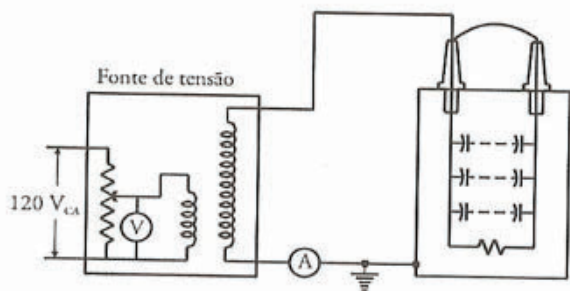
FIGURA – TESTE DE TENSÃO APLICADA VCA ENTRE OS TERMINAIS E A CAIXA
