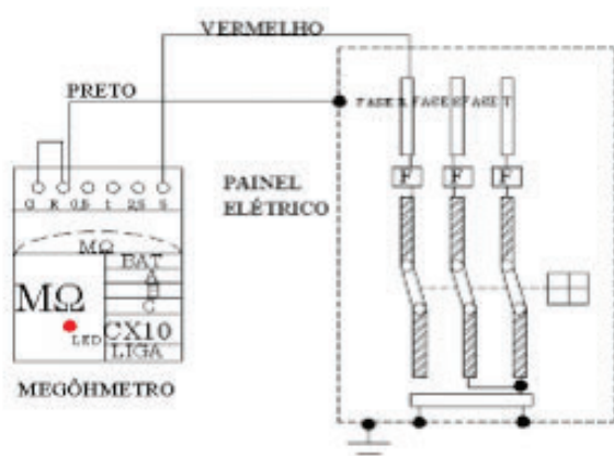
Figura 89: Ensaio de Resistência de Isolamento.
