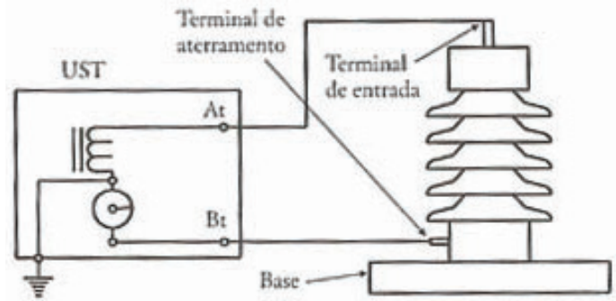
FIGURA– MEDIDA DE PERDAS DIELÉTRICAS EM UM PARA-RAIOS DE UMA UNIDADE
