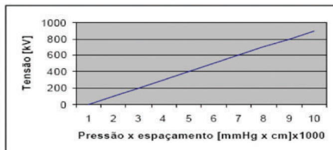
Figura 2 - Lei de Paschen para o ar com grandes vetores de "pd"
