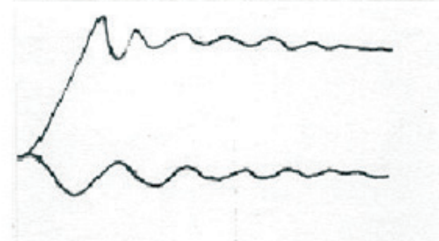
FIGURA 5 - Ligação Imprópria de Bobina
