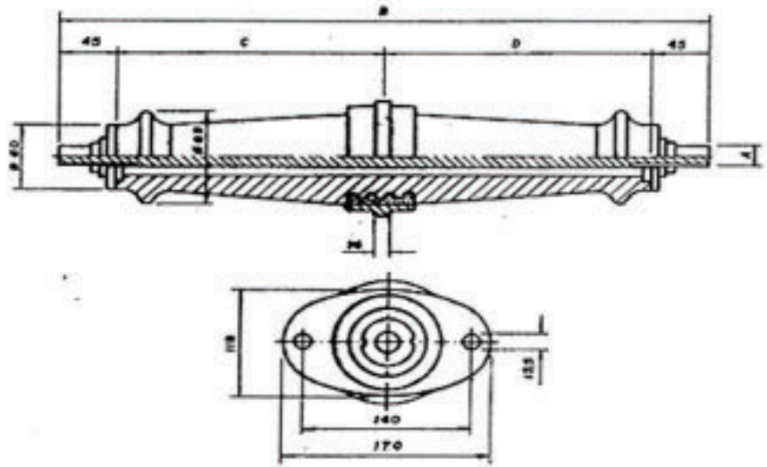
FIGURA 18 - ISOLADOR TIPO BUCHA DE PASSAGEM
