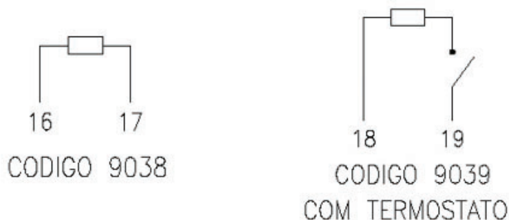
Figura 75: Resistência de Aquecimento
