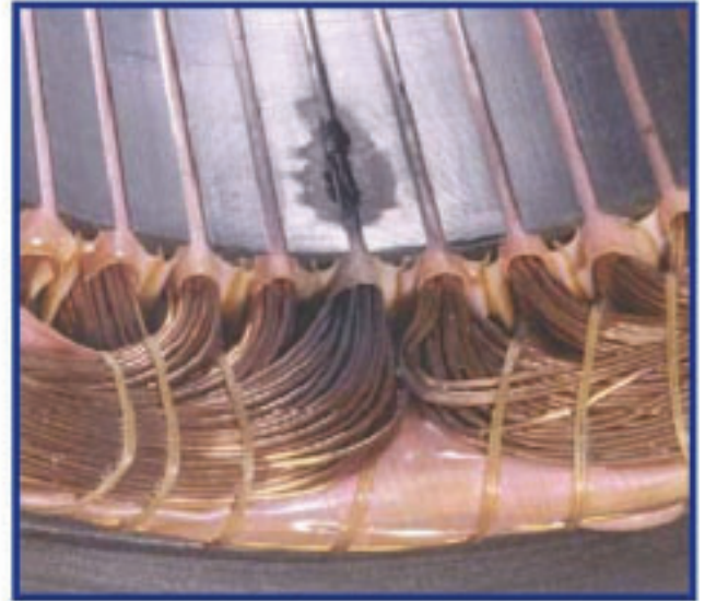
Figura 72: Curto contra a massa dentro da ranhura
