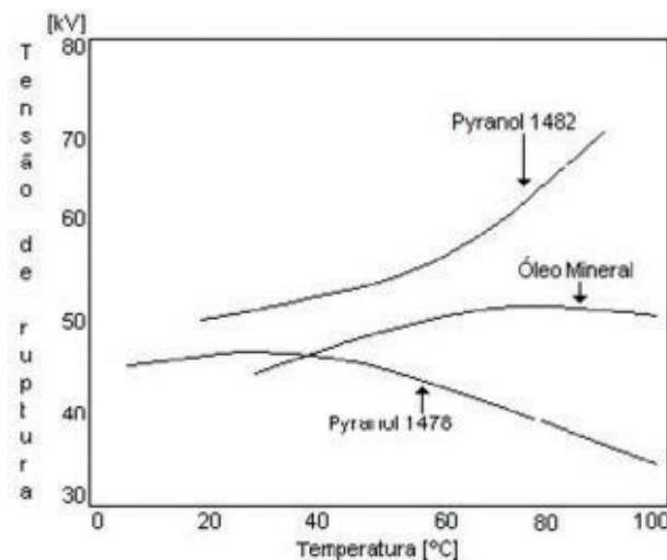
Figura 5 - Características de ruptura de óleos e pyrenol
