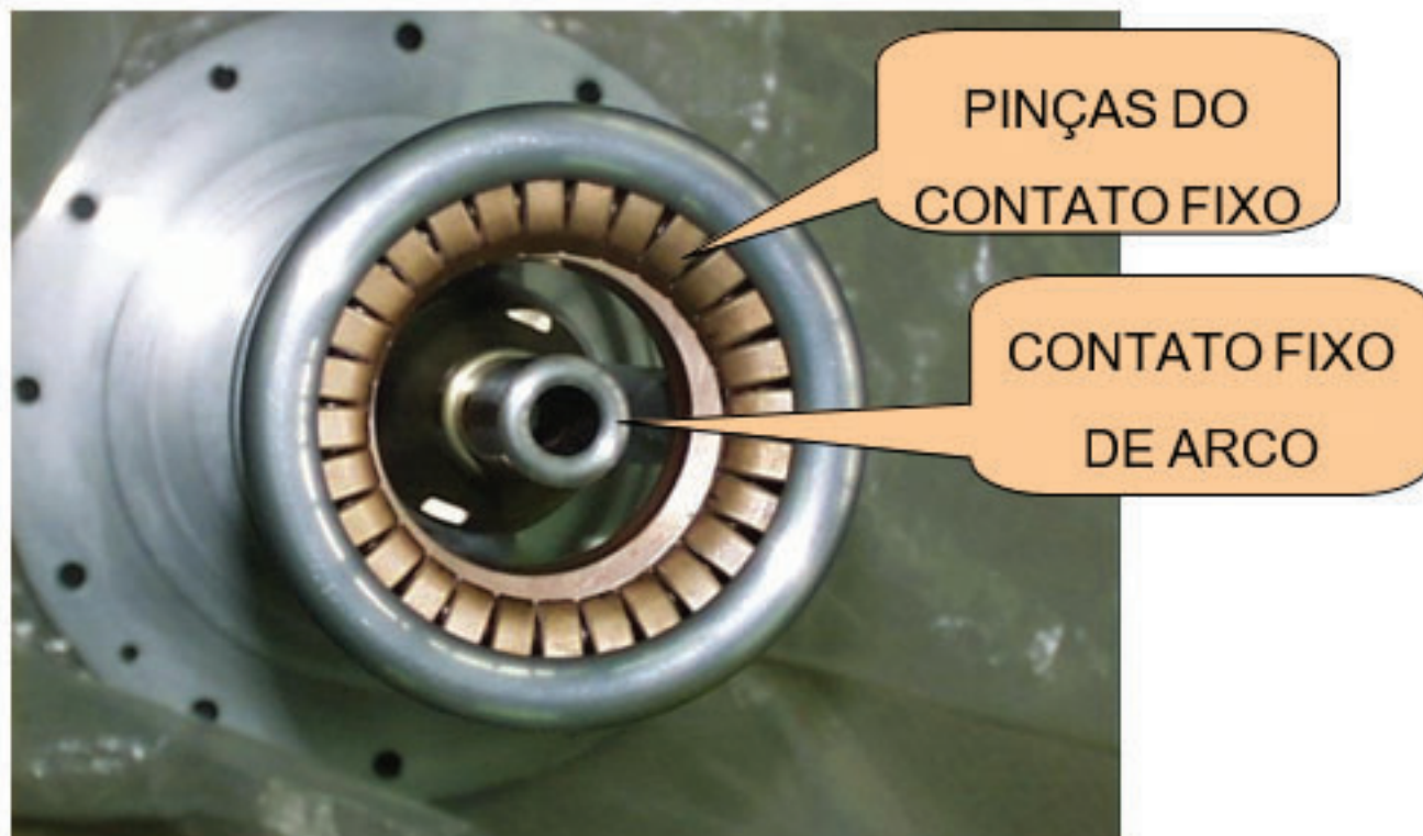
CONTATO DE ARCO
