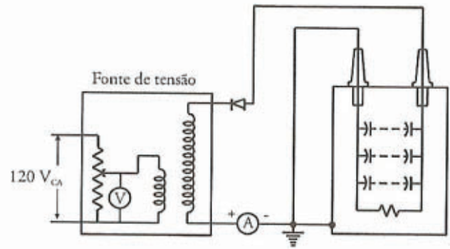
FIGURA – MEDIDA DA RESISTÊNCIA INTERNA DE CAPACITORES
