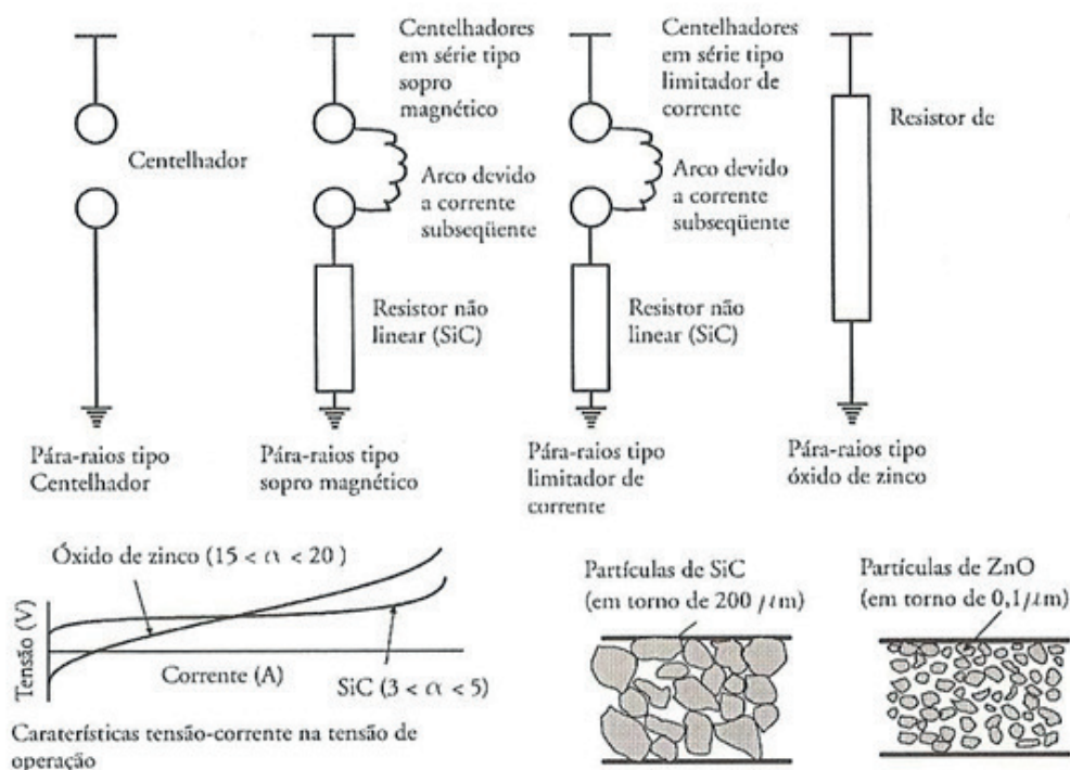
FIGURA – EVOLUÇÃO DA TECNOLOGIA DOS PARA-RAIOS
