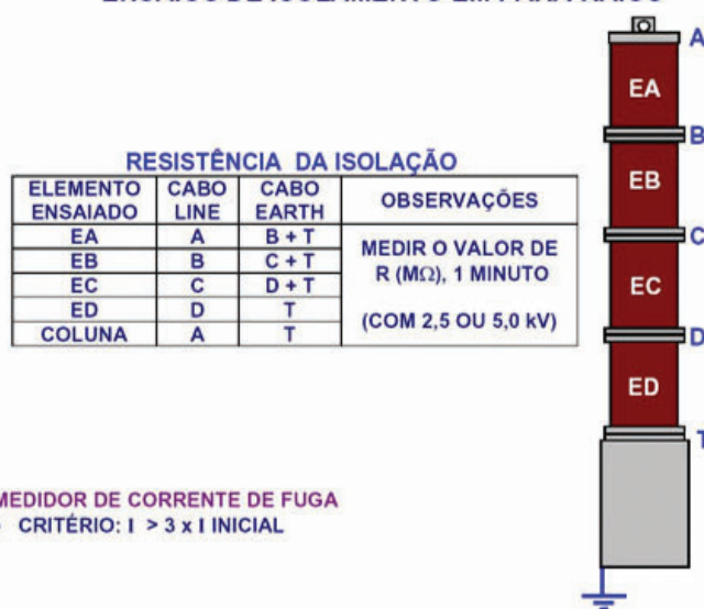
FIGURA – ENSAIO DE ISOLAMENTO
