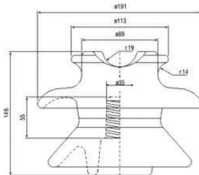
FIGURA 31 - SUPORTE TIPO PINO
