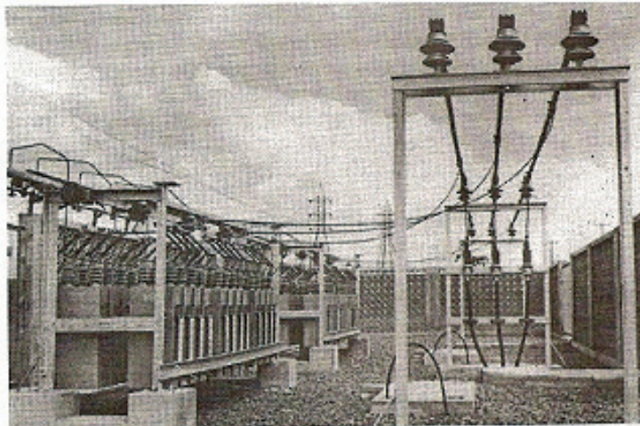
Figura 16.10.- Banco de capacitores sobre plataforma (rack) - Inducon
