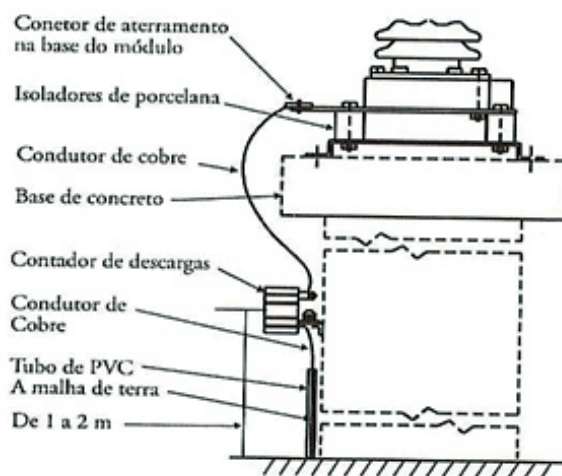
FIGURA – VISTA LATERAL DE UM PARA-RAIOS, COM CONTADOR DE DESCARGAS
