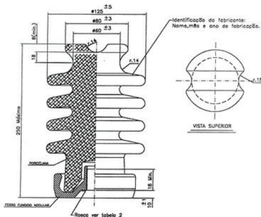
FIGURA 25 - ISOLADOR TIPO PILAR
