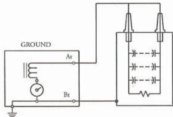
FIGURA– MEDIDA DO FATOR DE POTÊNCIA ENTRE OS TERMINAIS E CAIXA
