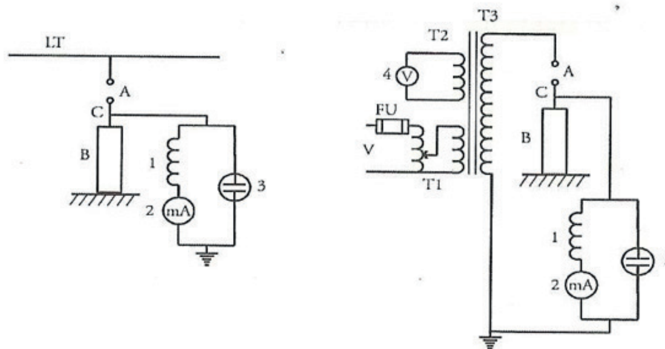
FIGURA – MEDIDA DE CORRENTE DE FUGA
