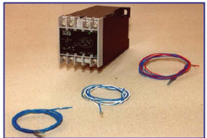
Figura 74: Termistores PTC
