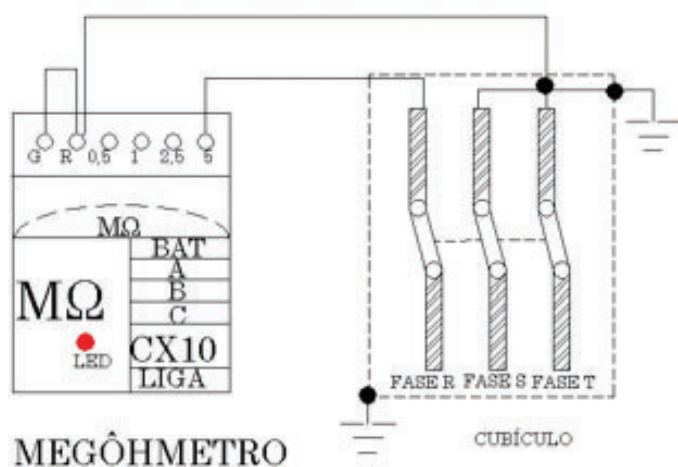
Figura 90: Ensaio de Resistência de Isolamento.
