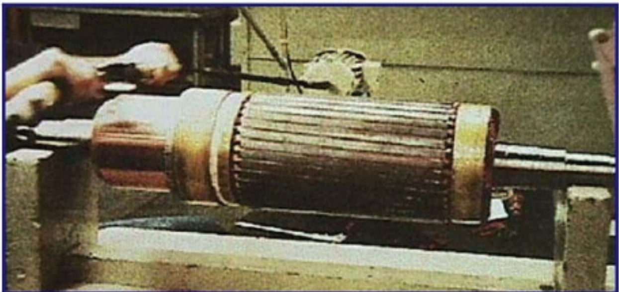
Figura 87: Isolação do comutador.
