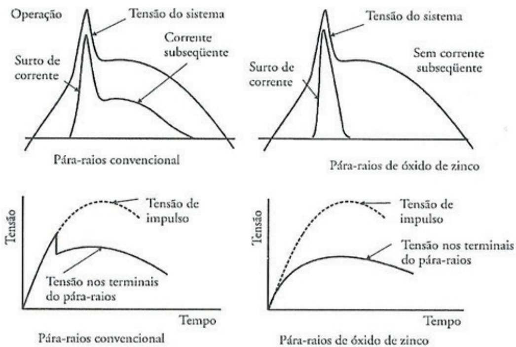
FIGURA – CARACTERÍSTICAS DE DESCARGA DE PARA-RAIOS CONVENCIONAIS E ZnO
