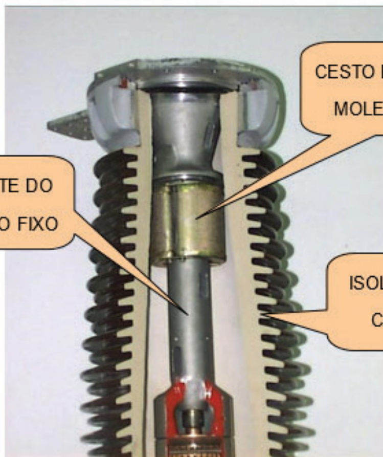
SUPORE DO CONTATO FIXO
