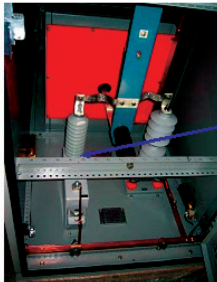
Figura 16.10.- Banco de capacitores sobre plataforma (rack) - Inducon
