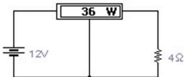
Figura 52: Wattímetro Digital
