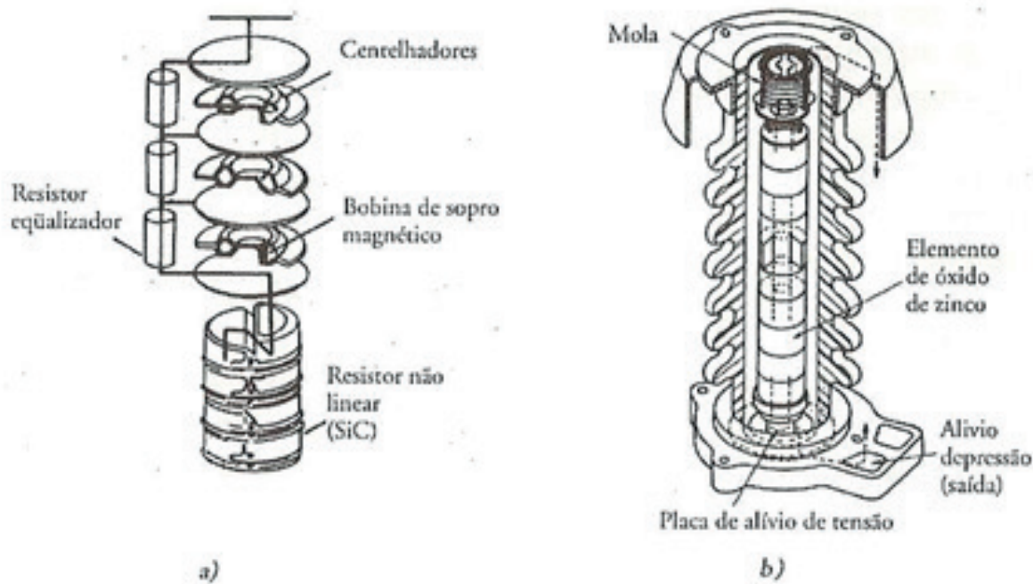
FIGURA – PARA-RAIOS: a) CONVENCIONAIS; b) DE ÓXIDO DE ZINCO
