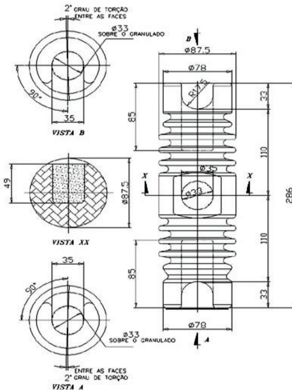
FIGURA 23 - ISOLADOR TIPO BUCHA PARA CHAVE FUSÍVEL
