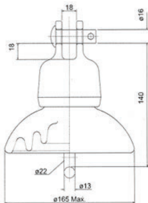
FIGURA 30 - ISOLADOR TIPO SUSPENSÃO
