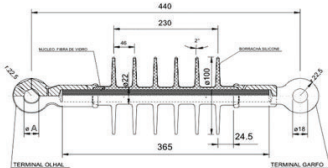
FIGURA 28 - ISOLADOR DE ANCORAGEM TIPO BASTÃO POLIMÉRICO
