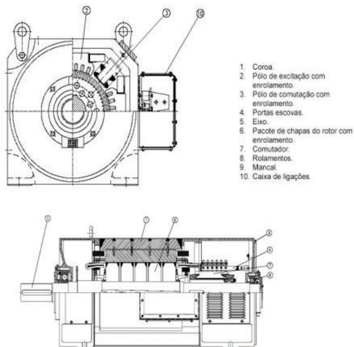
Figura 80: Partes construtivas de uma MCC.
