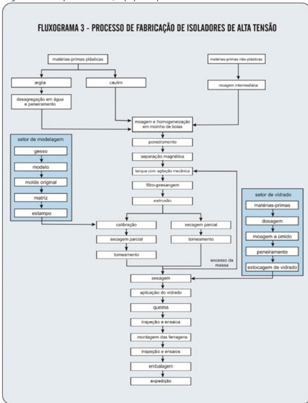
FIGURA16 - FLUXOGRAMA FABRICAÇÃO DE ISOLADORES DE ALTA TENSÃO
