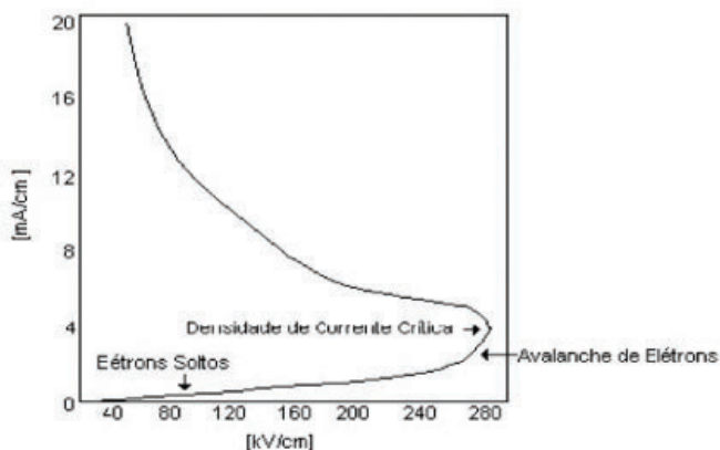
Figura 6 - características Volt-amperes de papel impregnado com óleo
