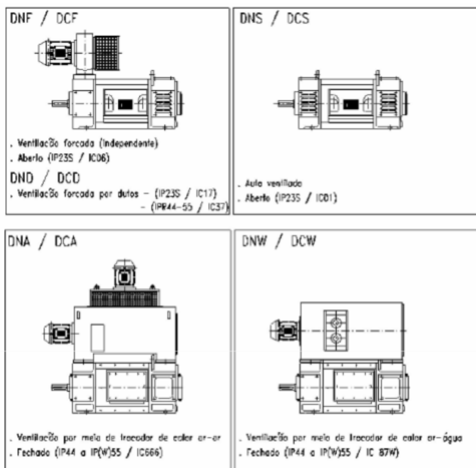
Figura 79: Tipos de ventilação.
