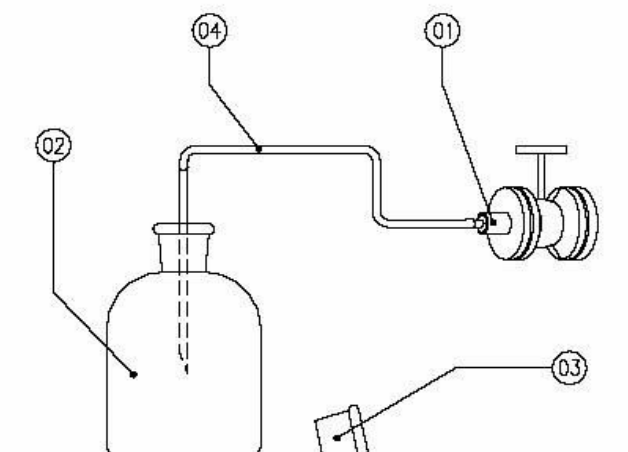
Figura 14 - Dispositivo para coleta de amostra de óleo para análise físico-química.
