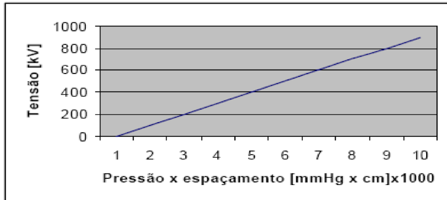
Figura 2 – Lei de Paschen para o ar com grandes valores de “pd”
