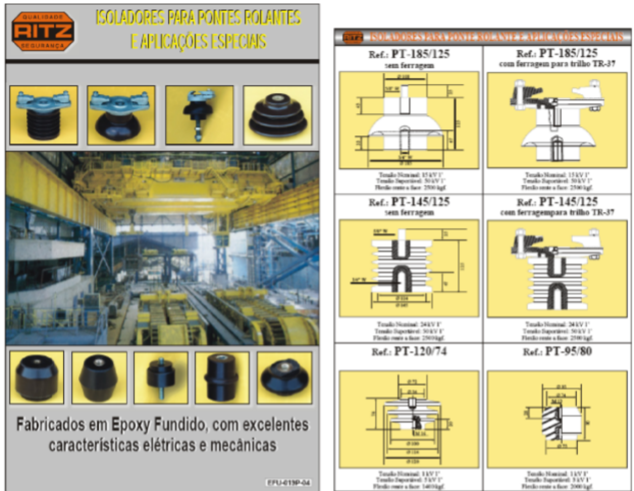
FIGURA 33 – ISOLADORES PARA PONTE ROLANTE E APLICAÇÕES ESPECIAIS
