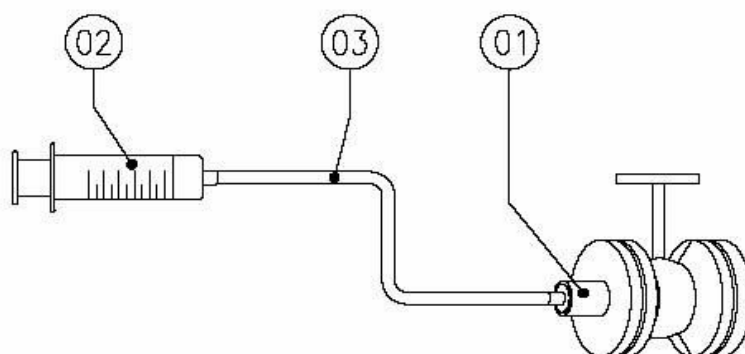
Figura 15 - Dispositivo para coleta de amostra de óleo para análise cromatográfica.
