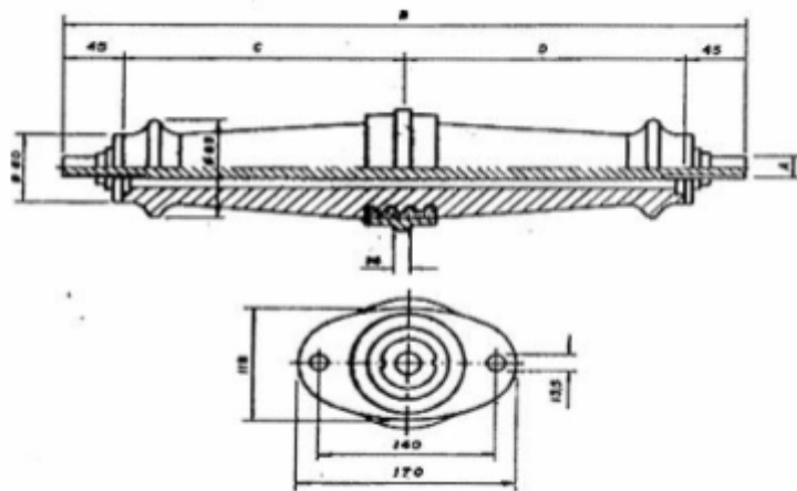
FIGURA 18 - ISOLADOR TIPO BUCHA DE PASSAGEM
