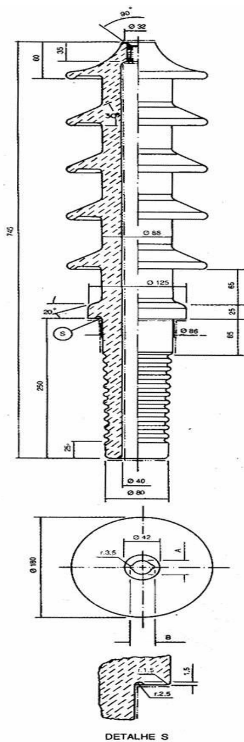
FIGURA 24 - ISOLADOR TIPO BUCHA TRAFO
