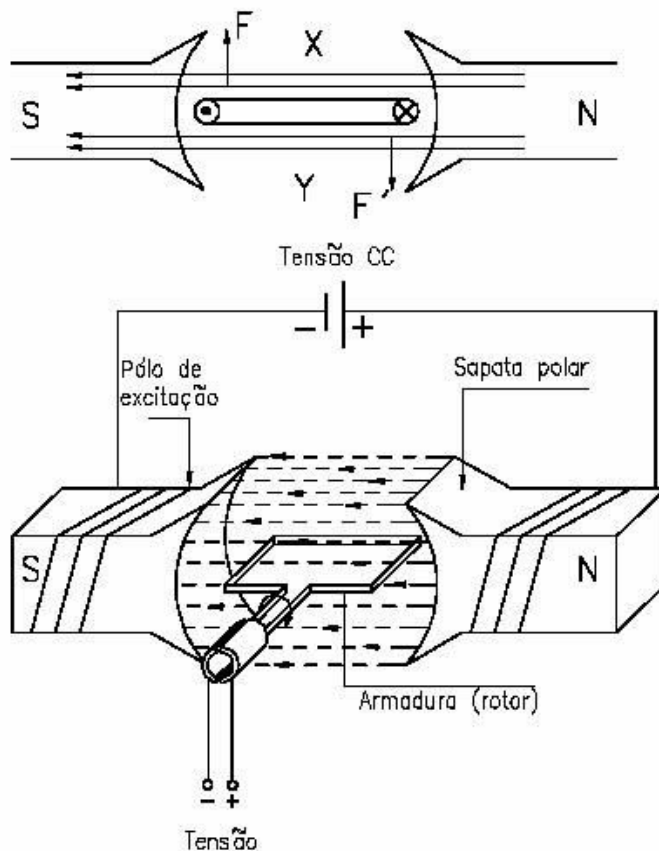
Figura 81: Princípios de funcionamento.
