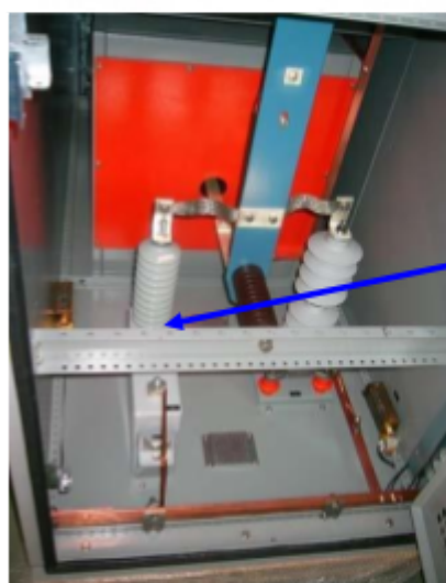
Figura 16.10.- Banco de capacitores sobre plataforma (rack) - Inducon
