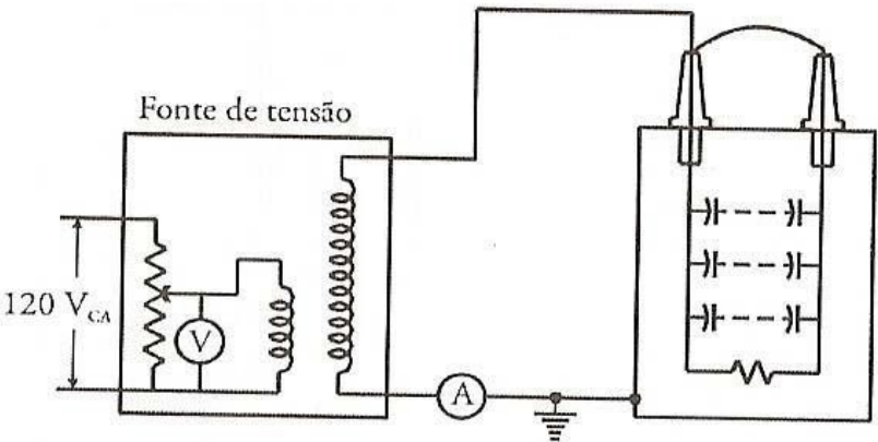
FIGURA– TESTE DE TENSÃO APLICADA VCA ENTRE OS TERMNAIS E A CAIXA
