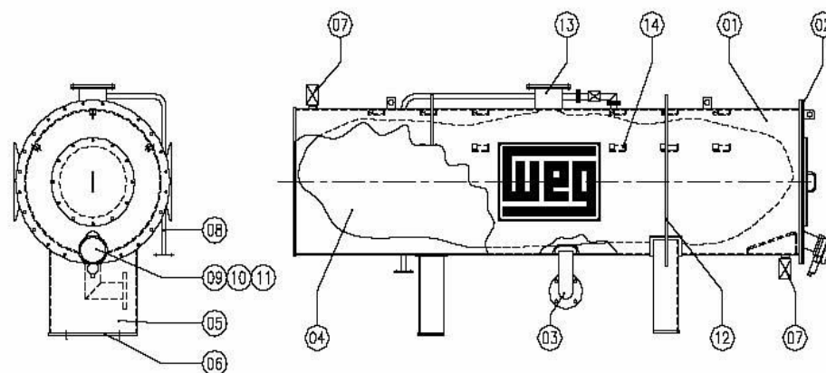
Figura 9 – Conservador de óleo com bolsa de borracha
