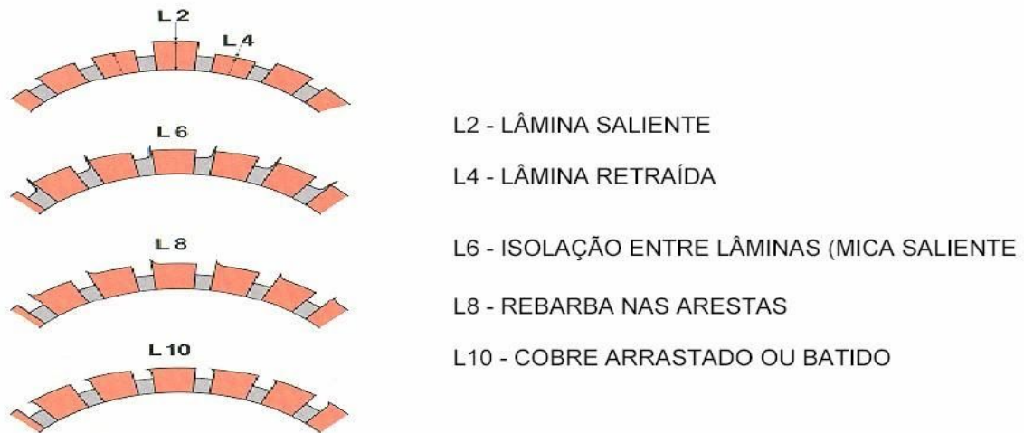
Figura 86: Defeitos na Lamelas.
