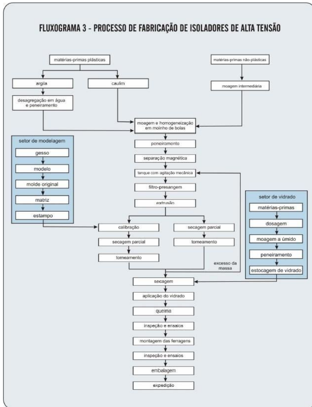
FIGURA - FLUXOGRAMA FABRICAÇÃO DE ISOLADORES DE ALTA TENSÃO
