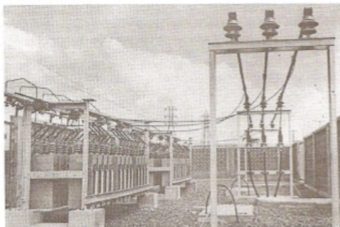
Figura 16.10.- Banco de capacitores sobre plataforma (rack) - Inducon
