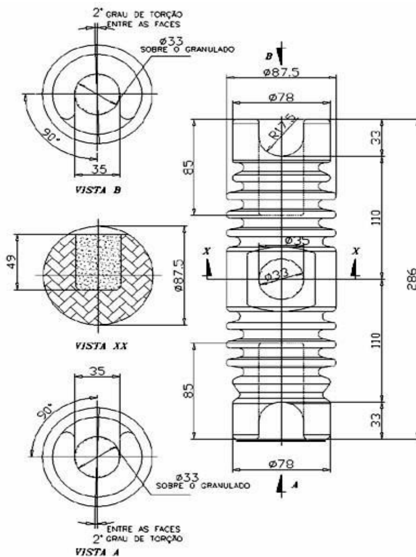
FIGURA - ISOLADOR TIPO BUCHA PARA CHAVE FUSÍVEL
