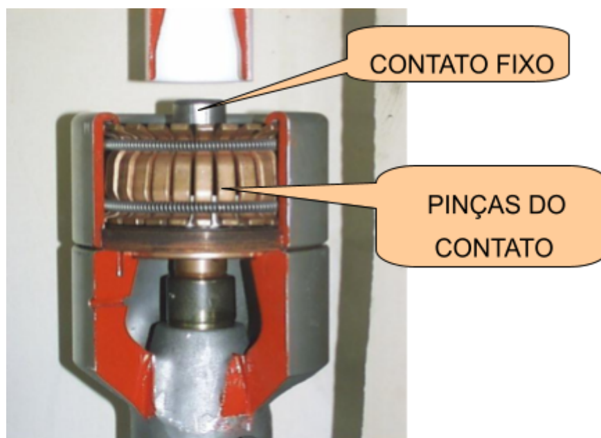
PINÇAS DO CONTATO FIXO
