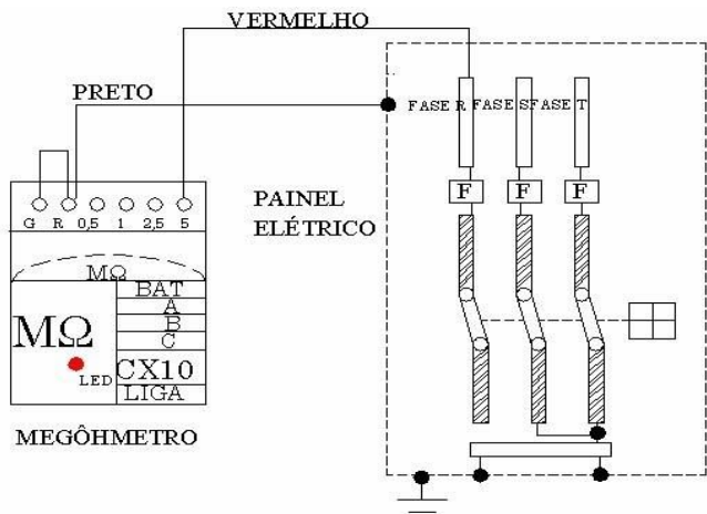
Figura 89: Ensaio de Resistência de Isolamento.
