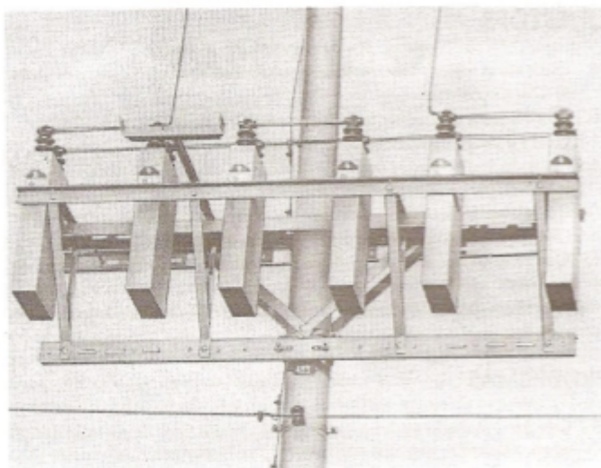
Figura 16.9.- Banco de capacitores sobre poste de concreto- Inducon
