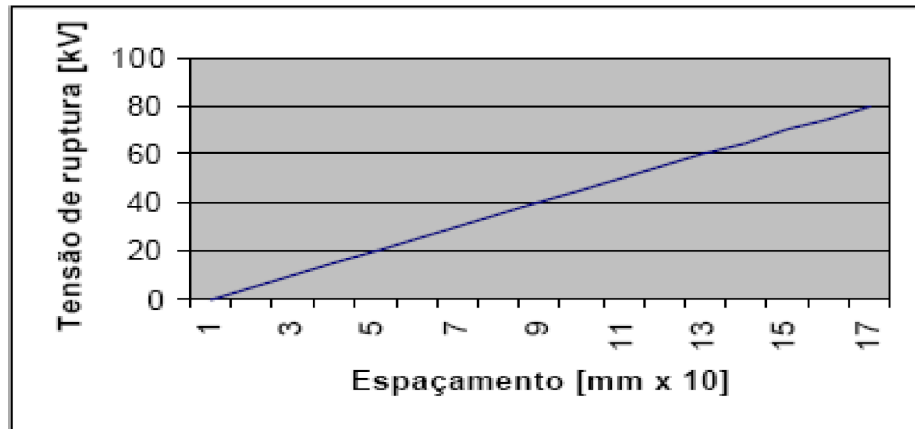
Figura 3 – Teste em óleo de grande pureza entre eletrodos esféricos
