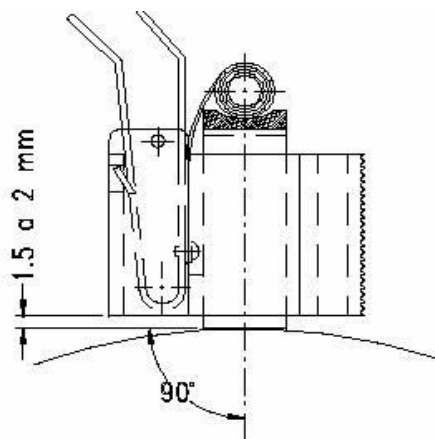
Figura 84: Porta Escovas.
