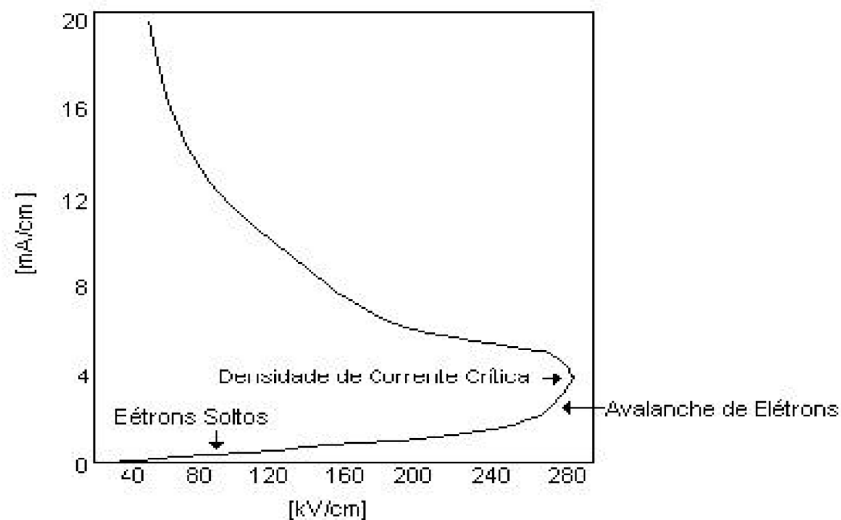
Figura 6 – Característica Volt-ampere de papel impregnado com óleo
