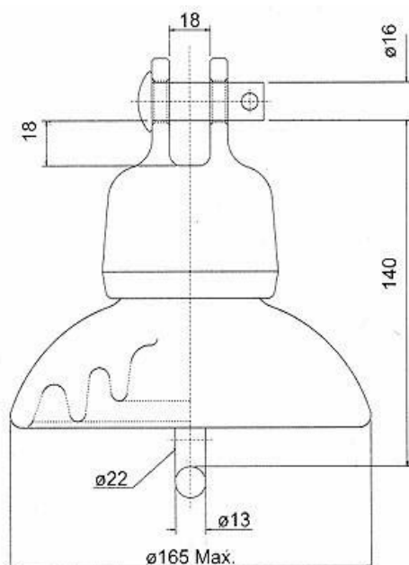
FIGURA 30 - ISOLADOR TIPO SUSPENSÃO FIGURA 31 - SUPORTE TIPO PINO
