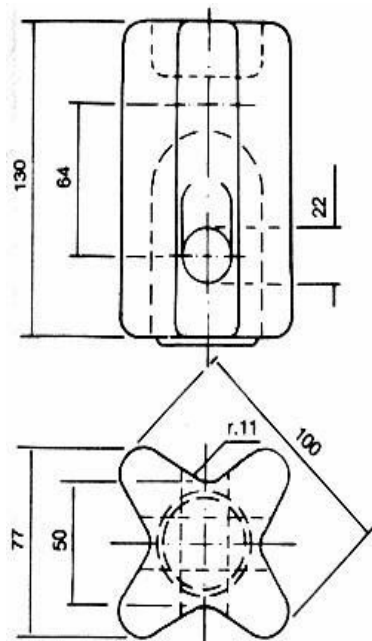
FIGURA 19 - ISOLADOR TIPO CASTANHA
