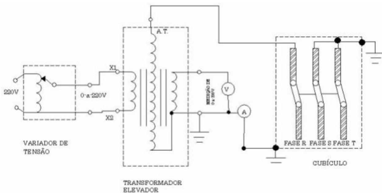
Figura 91: Ensaio de Tensão Aplicada.
