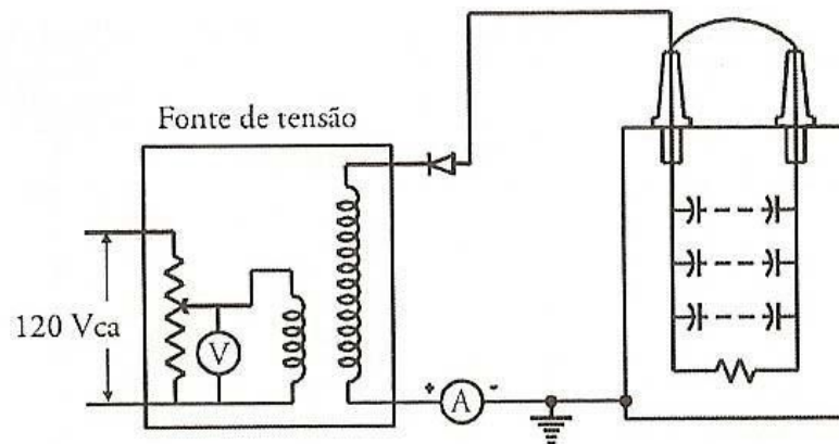
FIGURA – TESTE DE TENSÃO APLICADA VCC ENTRE OS TERMNAIS E A CAIXA
