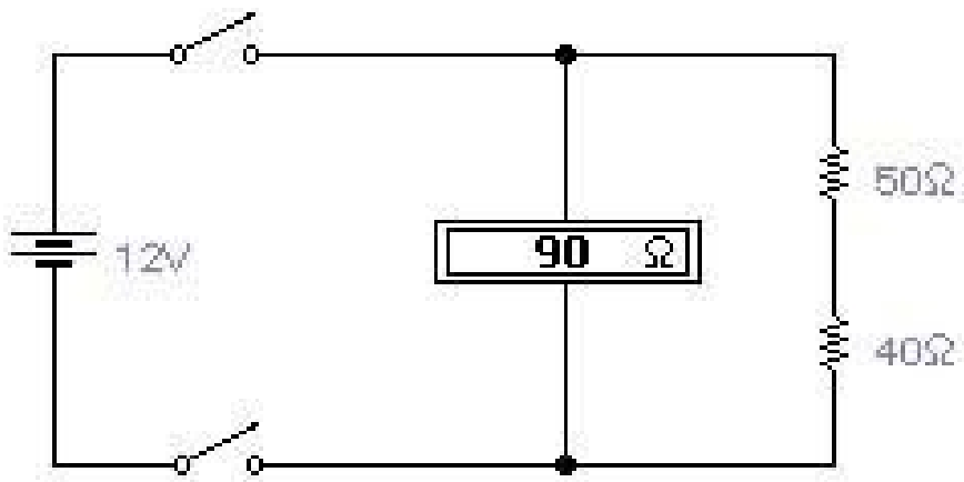
Figura 49: Medição Ohmímetro Digital
