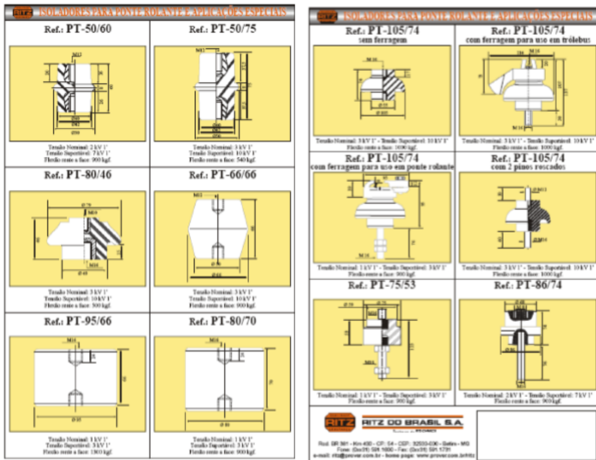
FIGURA 35 – ISOLADORES PARA PONTE ROLANTE E APLICAÇÕES ESPECIAIS
