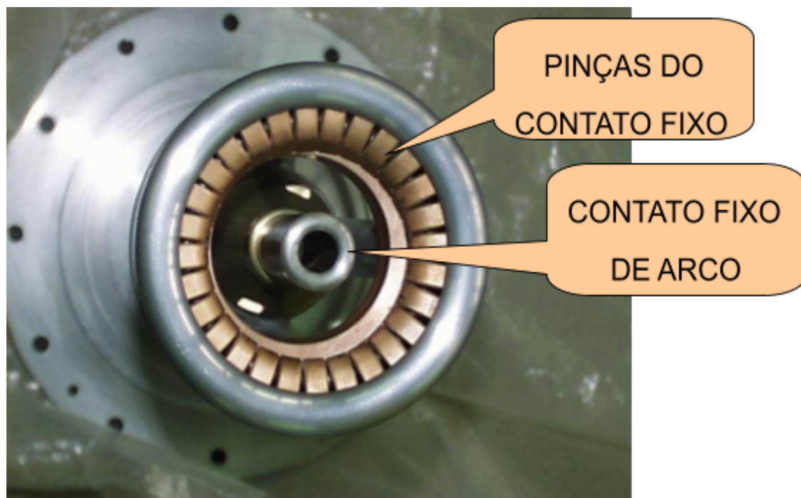
CONTATO FIXO DE ARCO
