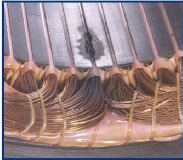
Figura 72: Curto contra a massa dentro da ranhura
