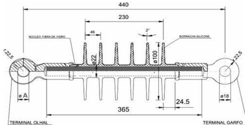
FIGURA 28 - ISOLADOR DE ANCORAGEM TIPO BASTÃO POLIMÉRICO
