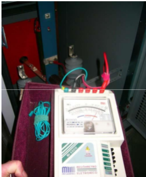
Figura 57: Megôhmetro Analógico de Alta Tensão - 5kv
