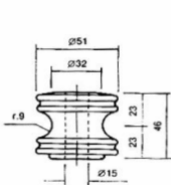
FIGURA 17 - ISOLADOR TIPO ROLDANA
