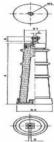
FIGURA 20 - ISOLADOR TIPO SUPORTE
