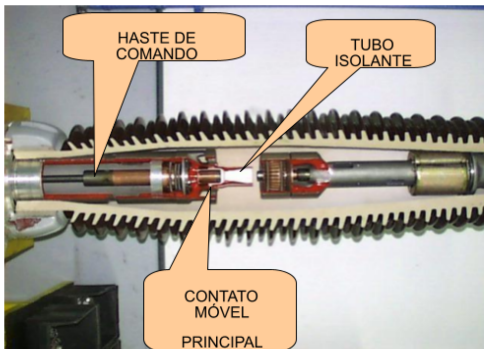
CORTE DA CÂMARA DE CONTATO
