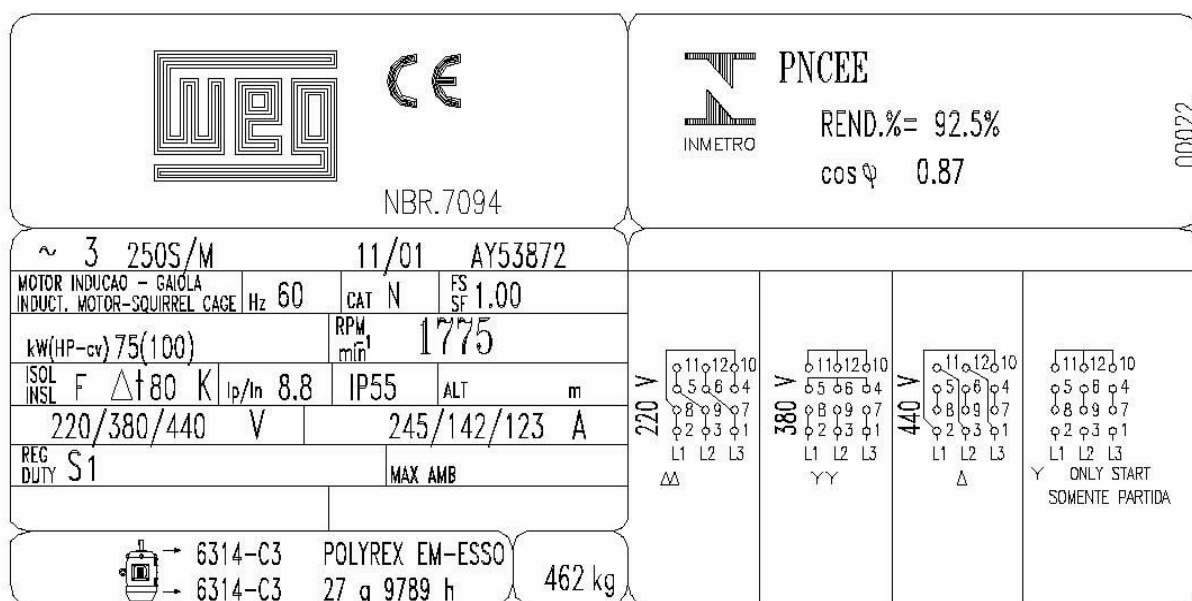
Figura 65: Placa e Identificação de Motor Trifásico
