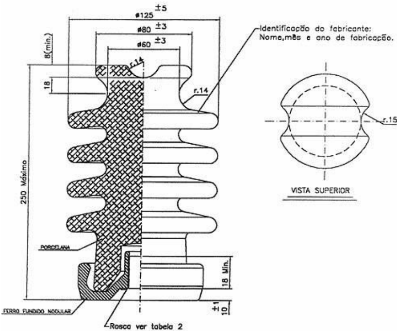
FIGURA 25 - ISOLADOR TIPO PILAR
