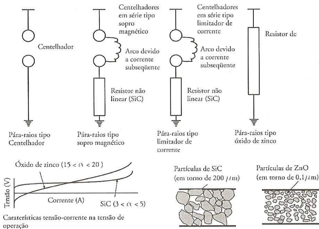
FIGURA– EVOLUÇÃO DA TECNOLOGIA DOS PARA-RAIOS
