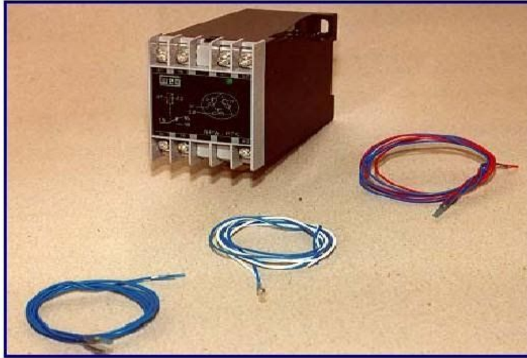
Figura 74: Termistores PTC
