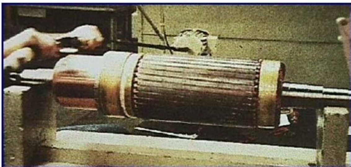
Figura 87: Isolação do comutador.
