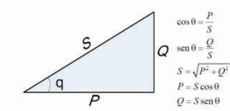
Figura – Triângulo das Potências
