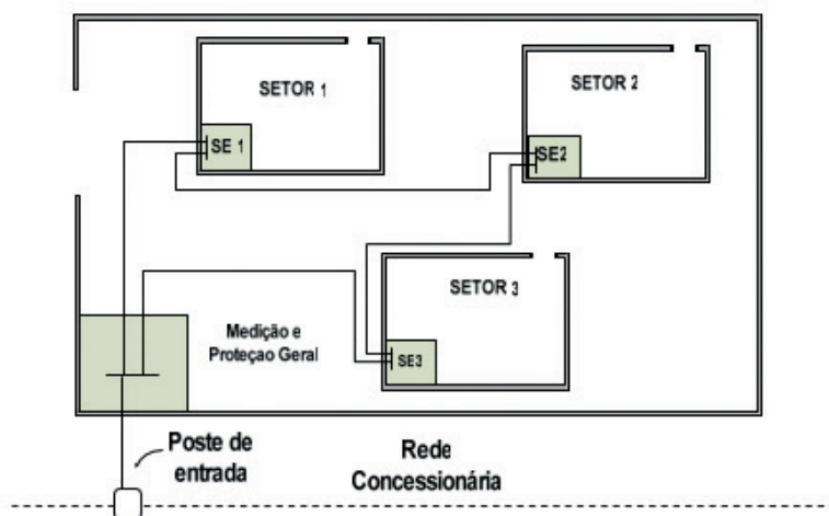
Figura – Sistema radial com recurso
