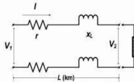
(b) Circuito elétrico monofásico equivalente
