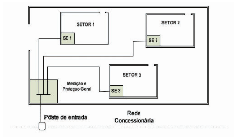
Figura – Sistema radial simples
