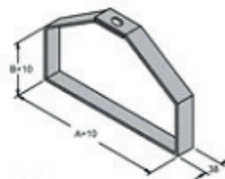
Código: PL 1139 Suporte vertical tipo "B"
