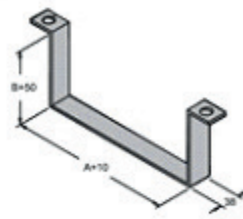
Código: PL 1129 Suporte ômega
