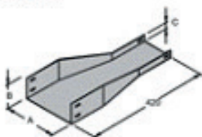
Código: PL 190 Redução de abas
