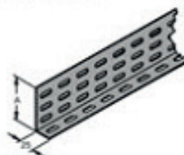
Código: PL 14190 Septo divisor perfurado
