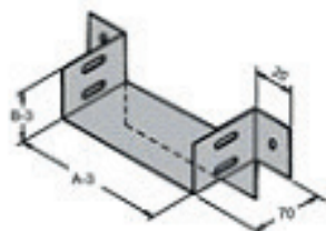
Código: PL 1109 Flange para ligação em painel
