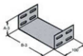
Código: PL 100 Emenda interna "U"
