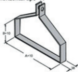
Código: PL 1119 Suporte horizontal tipo "A"
