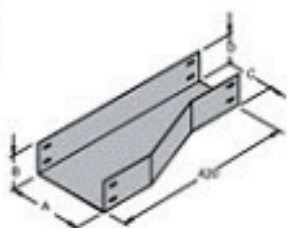
Código: PL 189 Redução a esquerda
