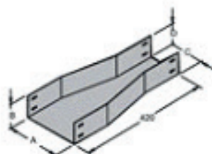
Código: PL 199 Redução concêntrica
