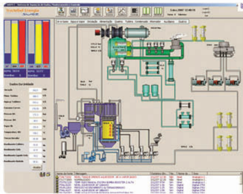
Figura: Tela de visão geral do processo
