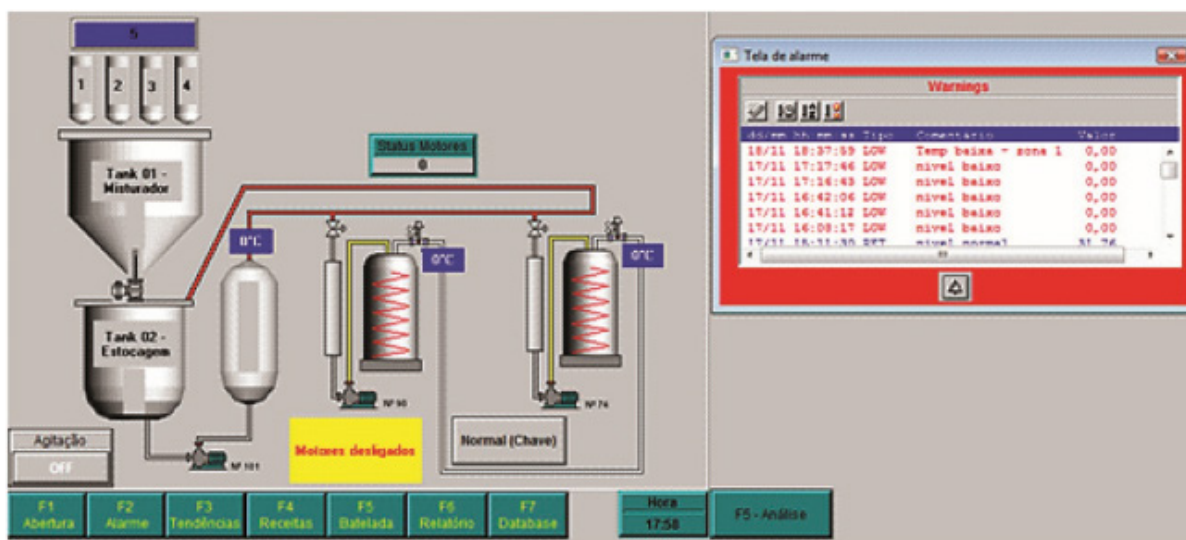
Figura: Exemplo de tela de manutenção
