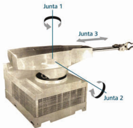
Figura: Unimate, o primeiro robô industrial
