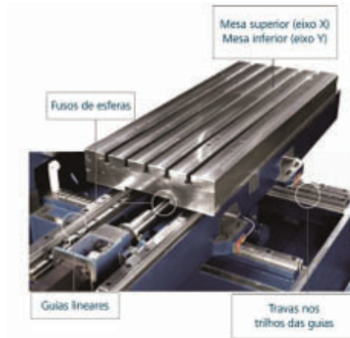
Figura: Conjunto de movimentação e apoio
