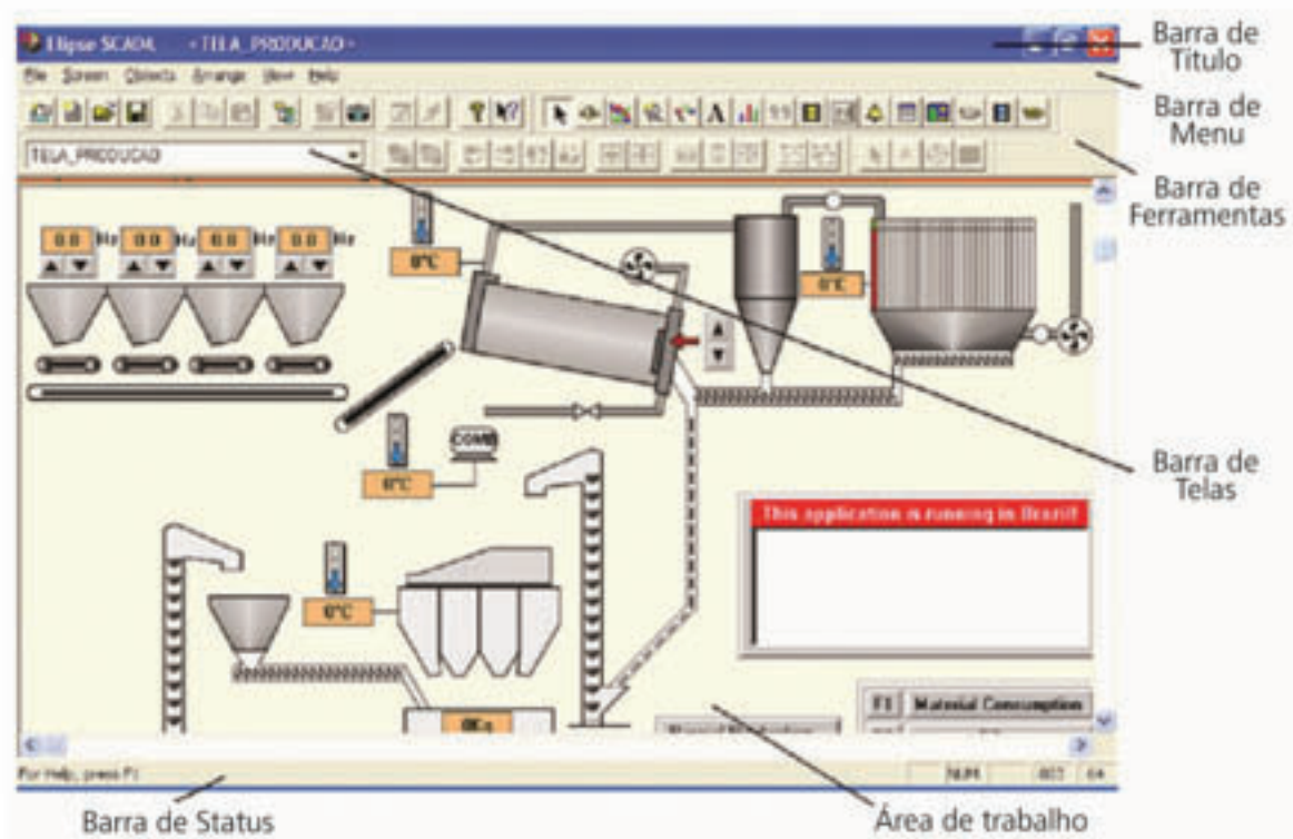
Figura: Tela principal do SCADA quando uma aplicação está aberta, no módulo configurador, identificando seus elementos
