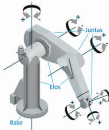
Figura: Componentes de um robô industrial
