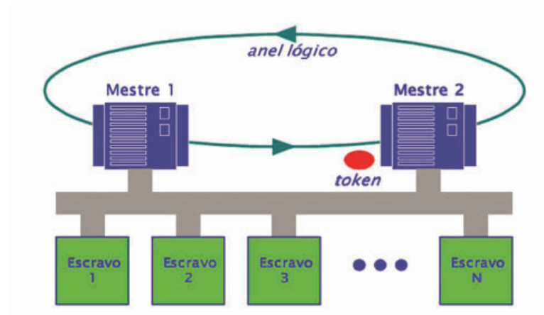
Figura: Exemplo de aplicação do protocolo Profibus
