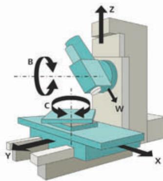
Figura: Máquina-ferramenta com seis eixos coordenados
