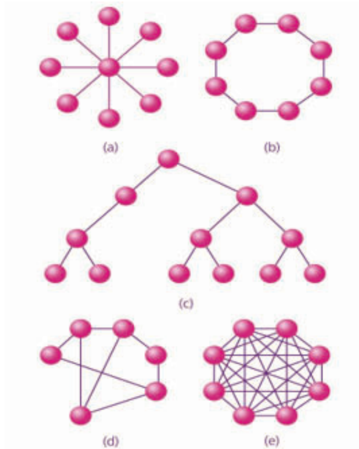
Figura: Topologias de redes ponto-a-ponto: (a) estrela, (b) anel, (c) árvore, (d) malha regular e (e) malha irregular
