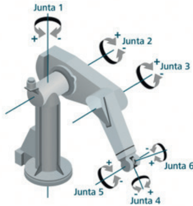
Figura: Robô articulado com 6 graus de liberdade
