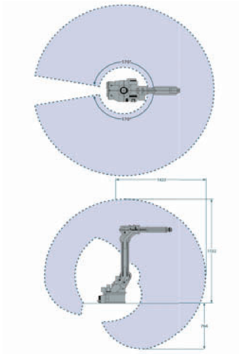
Figura: Espaço de trabalho do robô Motoman MH6-S
