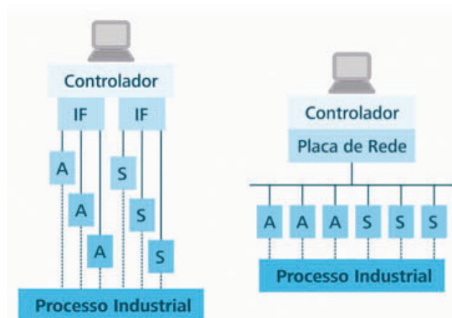
Figura: Diferenças básicas entre um sistema de controle tradicional e um sistema de controle com Fieldbus
