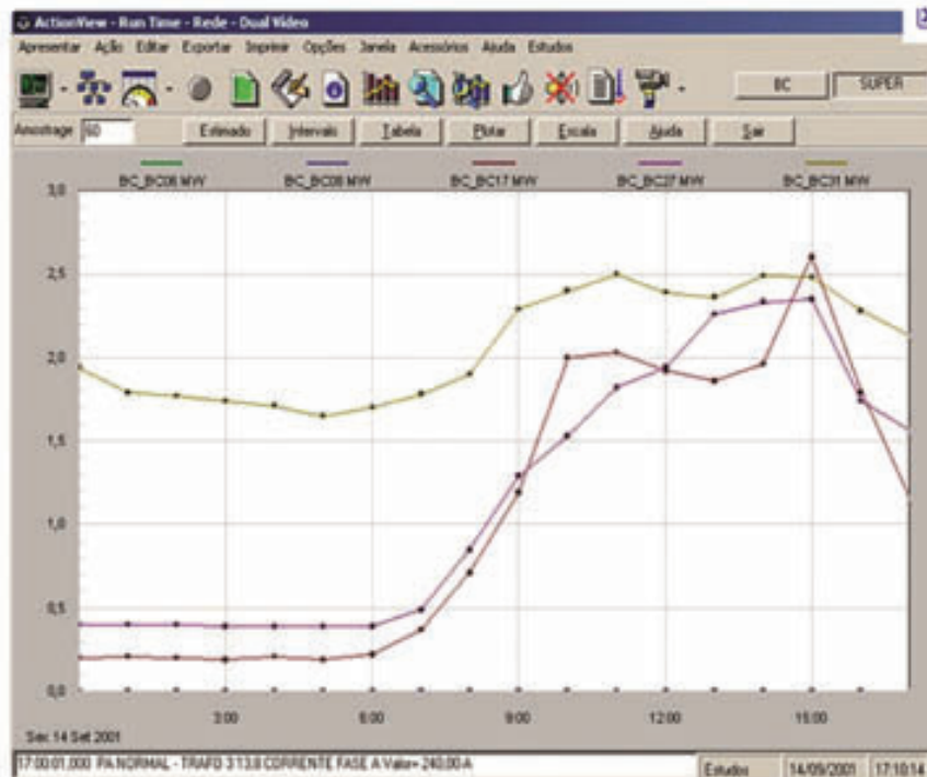
Figura: Exemplo de tela de tendência
