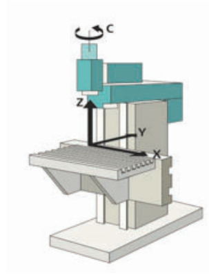
Figura: Máquina-ferramenta com três eixos coordenados
