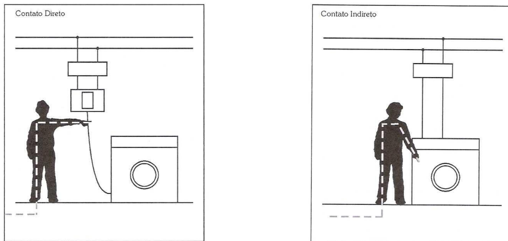
Figura - Choque elétrico por contato direto e indireto.
