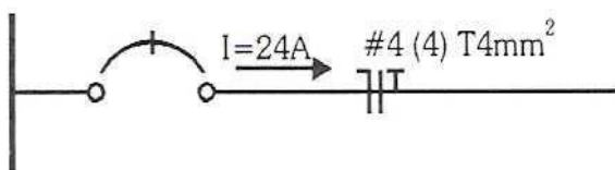
Figura - Exemplo de dimensionamento de dispositivo de proteção.
