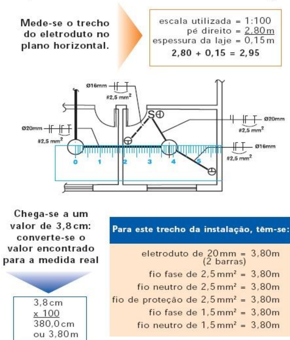
Figura– Exemplo do levantamento de eletrodutos e da fiação.
