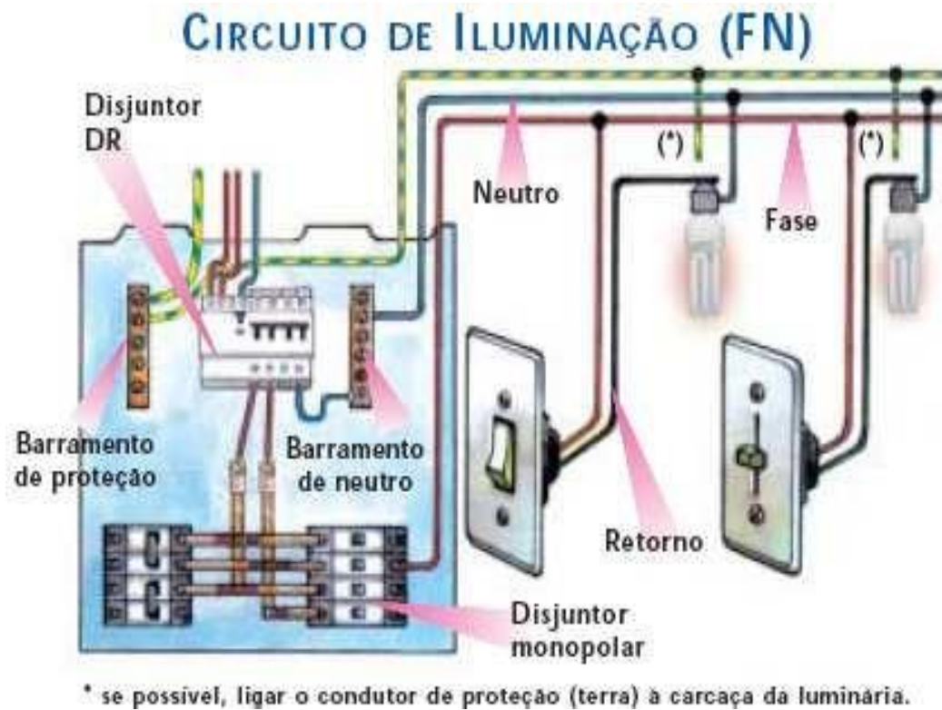
Figura - Circuito de iluminação fase-neutro
