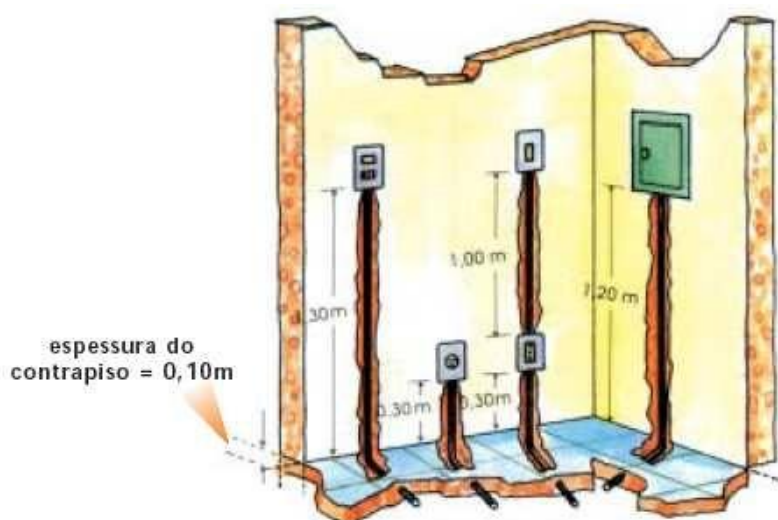
Figura– Medidas dos eletrodutos que sobem até as caixas.
