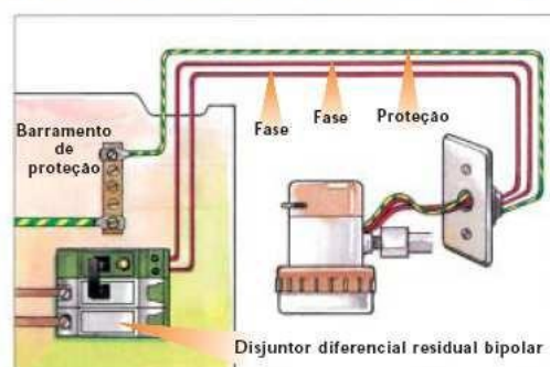
CIRCUITO DE TOMADA DE USO ESPECÍFICO (FF)
