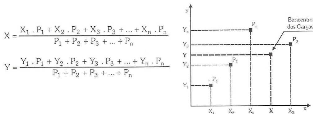
Figura - Cálculo do centro das cargas.
