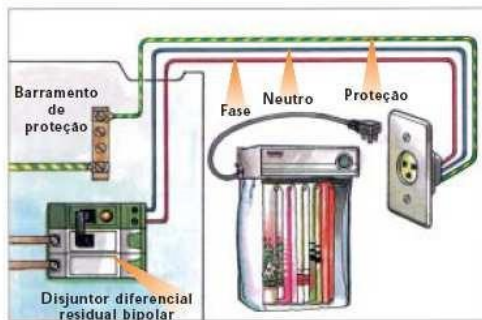
CIRCUITO DE TOMADA DE USO ESPECÍFICO (FN)
