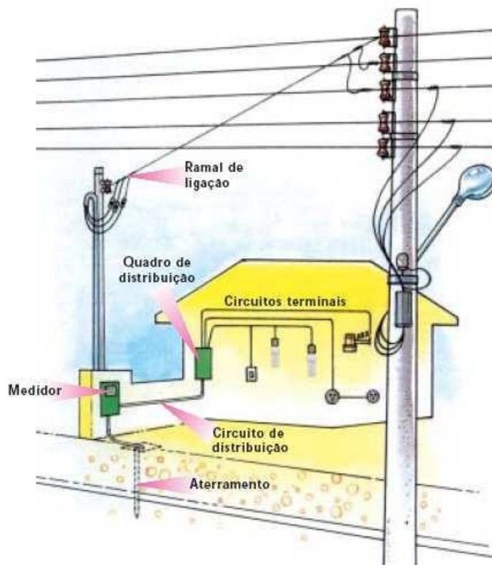
Figura (c) Rede pública de baixa tensão
