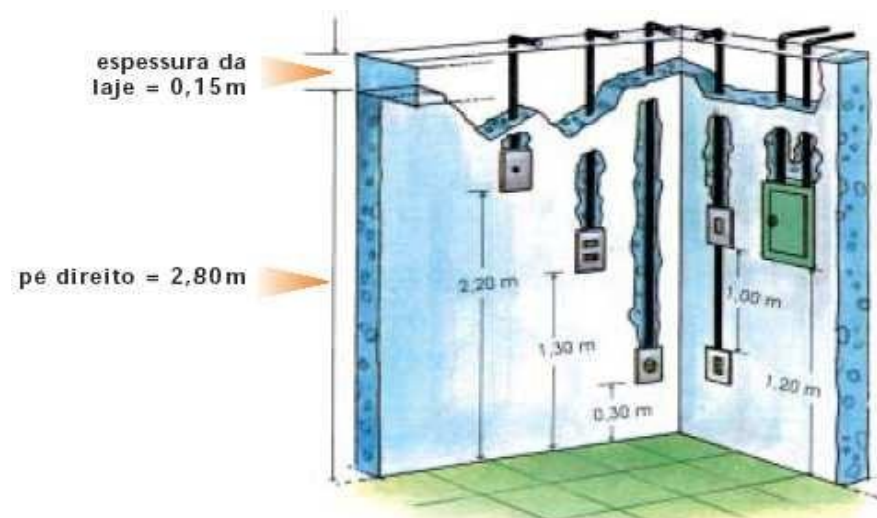
Figura– Medidas dos eletrodutos que descem até as caixas.
