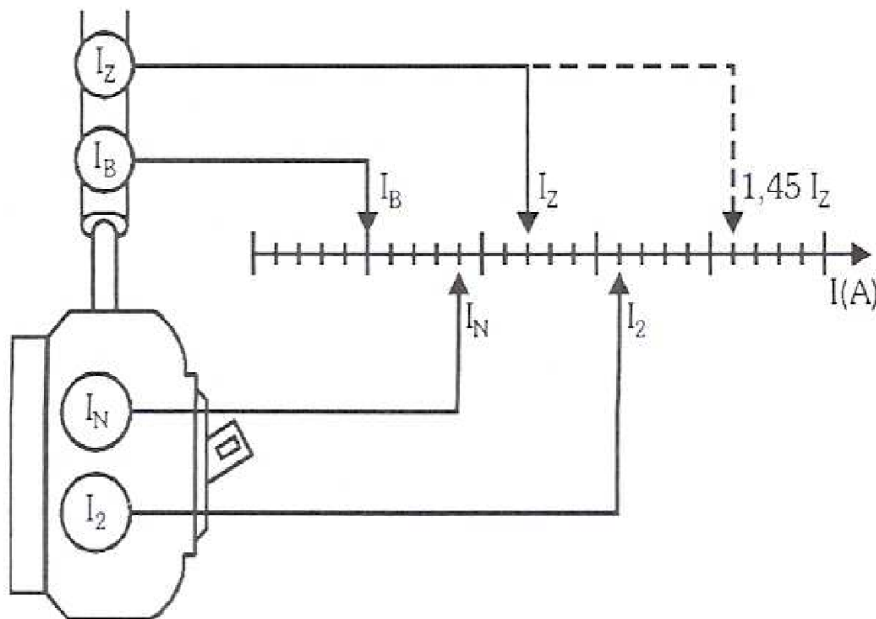
Figura - Condições de proteção contra sobrecargas.
