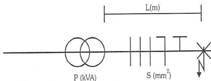
Figura Curto-circuito em um alimentador trifásico.
