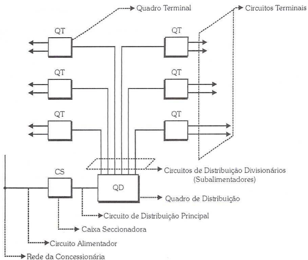
Figura - Circuitos de distribuição e circuitos terminais.
