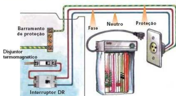
CIRCUITO DE TOMADA DE USO ESPECÍFICO (FN)
