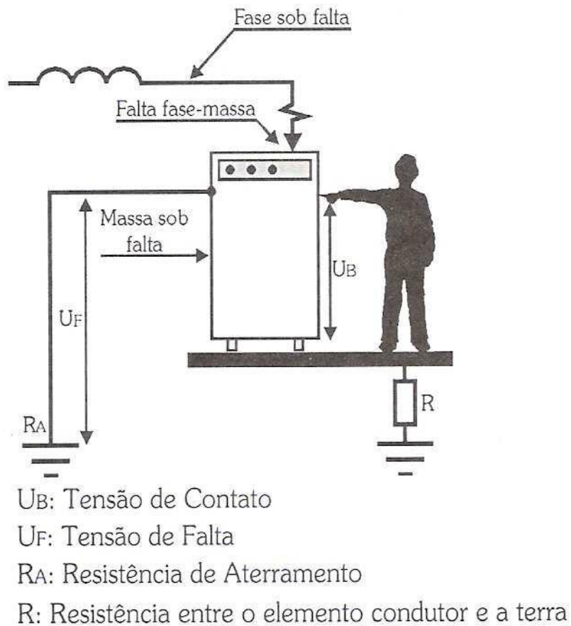
Figura - Tensão de contato e tensão de falta.
