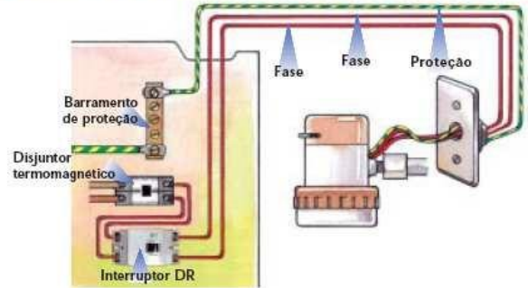
CIRCUITO DE TOMADA DE USO ESPECÍFICO (FF)
