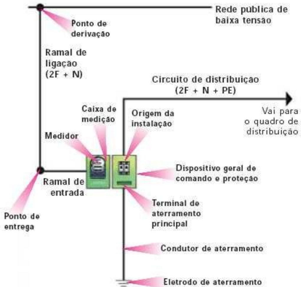
Figura - Circuito de distribuição, caixa de medição e quadro de distribuição.
