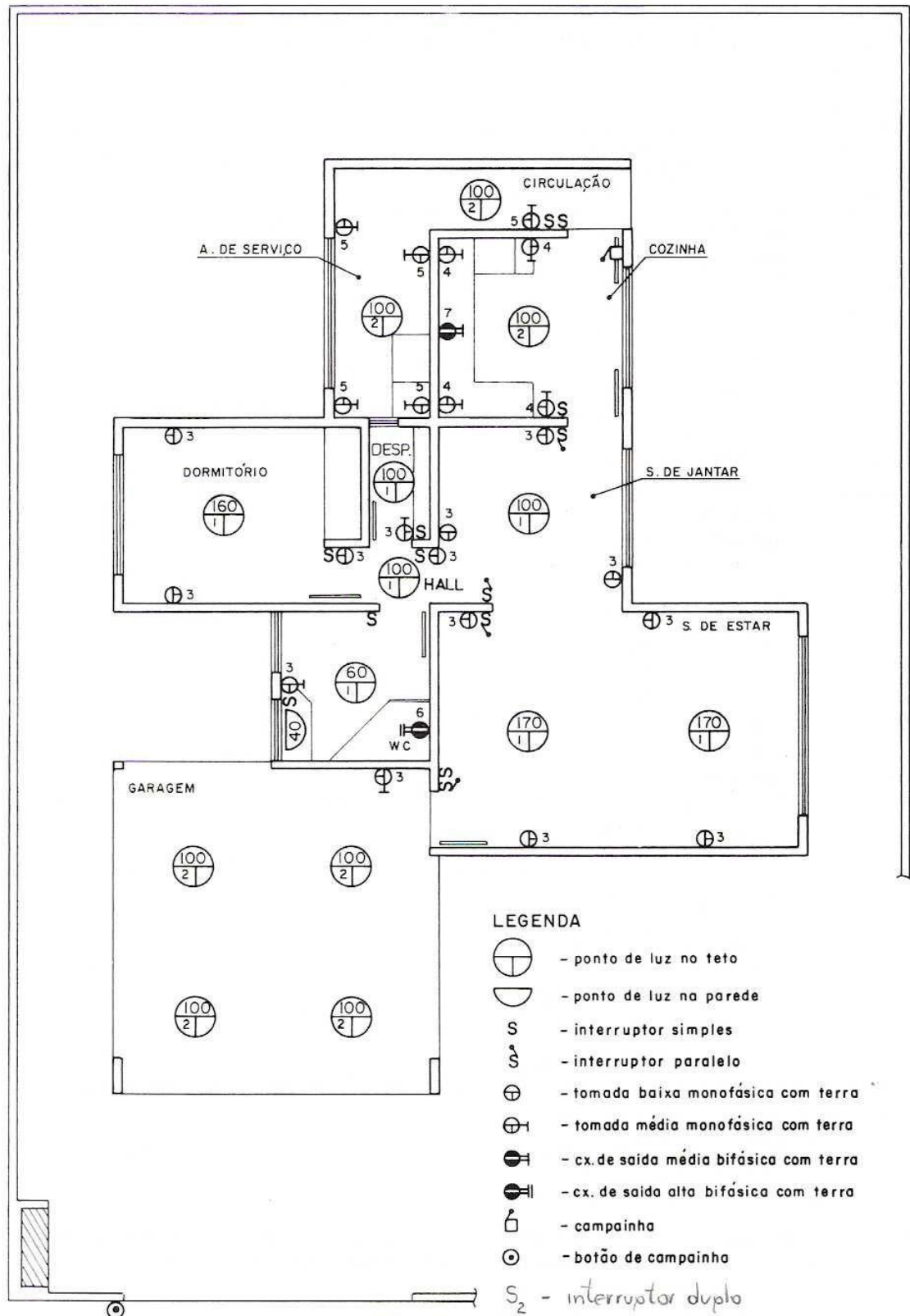
Figura - Indicando na planta o número do circuito.
