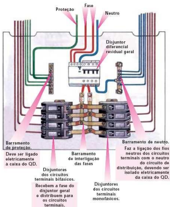
Figura - Exemplo de quadro de distribuição para fornecimento bifásico.
