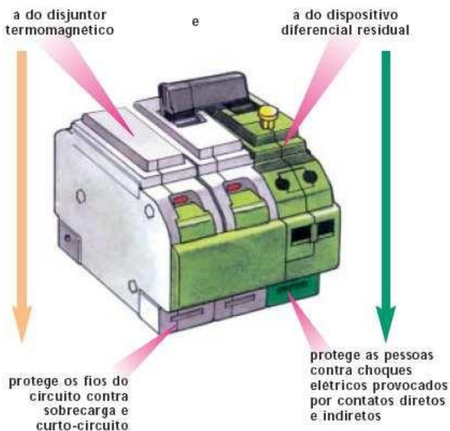
Figura - Disjuntor diferencial residual
