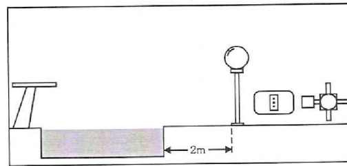
Figura – Instalação de dispositivos DR's.
