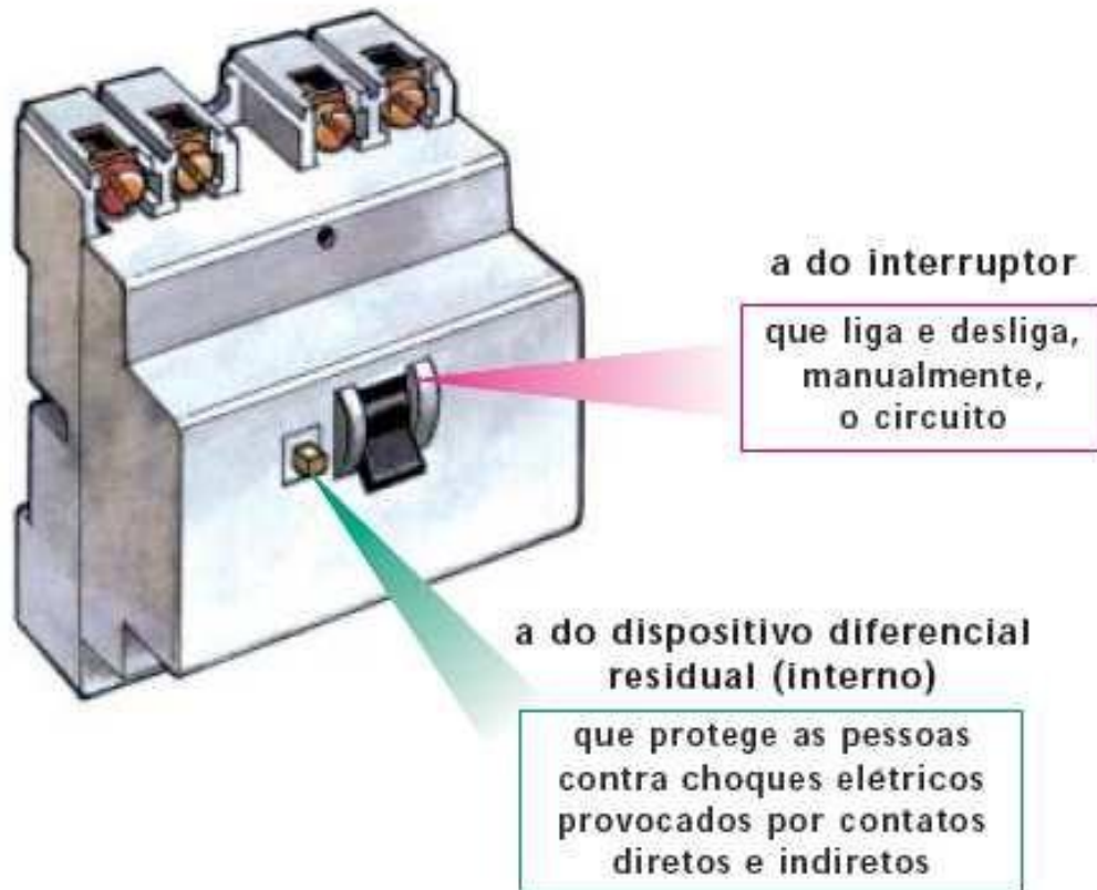
Figura -. Interruptor diferencial residual
