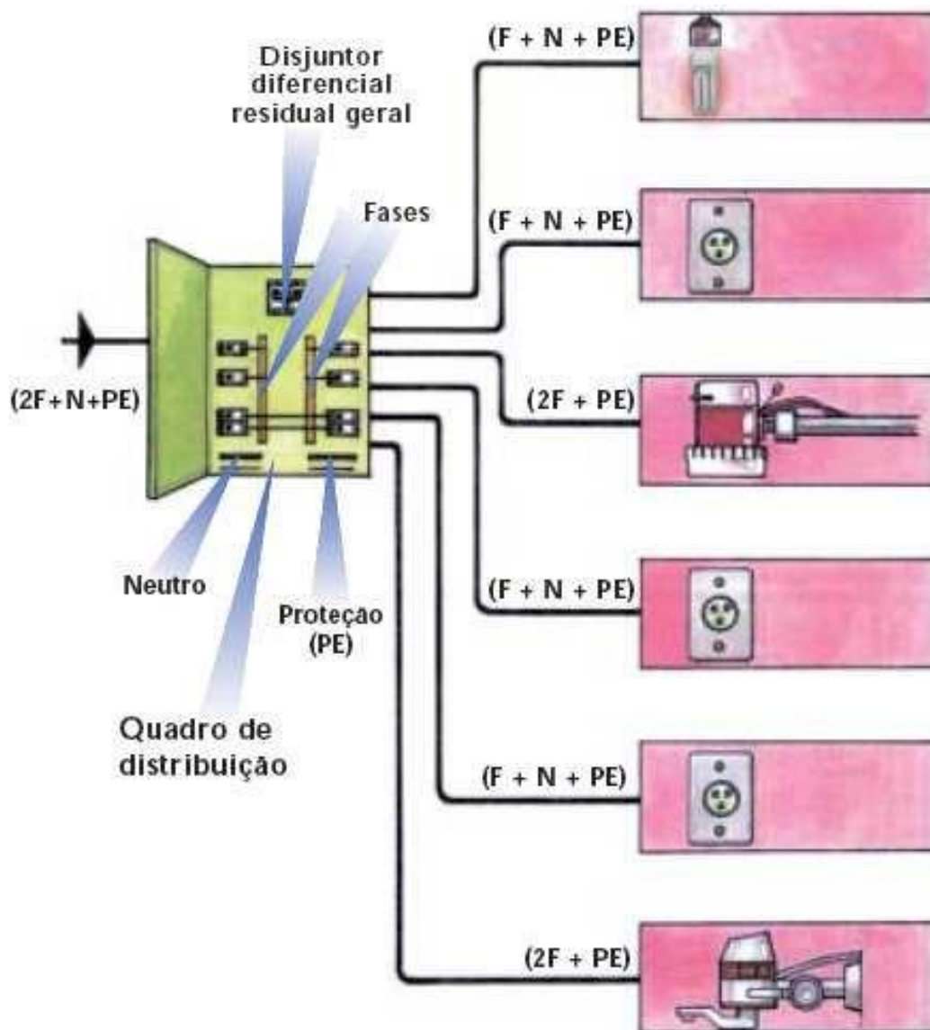
Figura -Circuitos terminais de uma instalação residencial.
