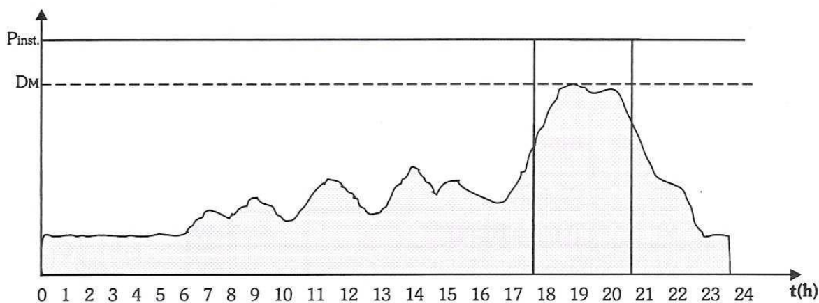
Figura - Exemplo de curva de solicitação diária de um consumidor residencial.
