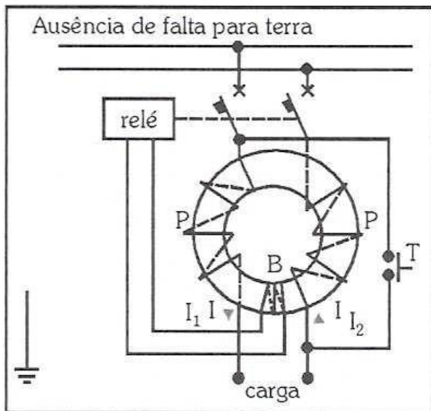
Figura – Funcionamento elétrico de um dispositivo DR.
