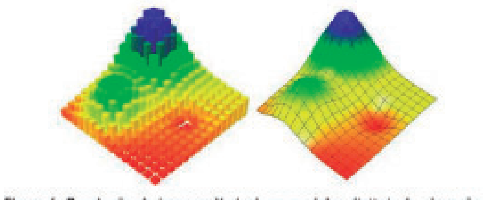
Figura 6. Resolução da imagem X pixel em modelos digitais de elevação
