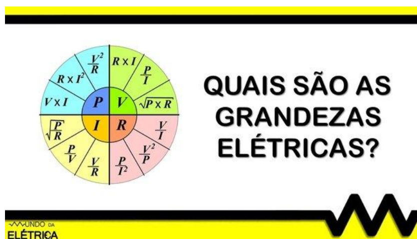
Figura 1: Grandezas elétricas.
