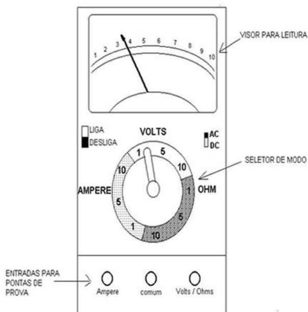
Figura 3: Multímetro.
