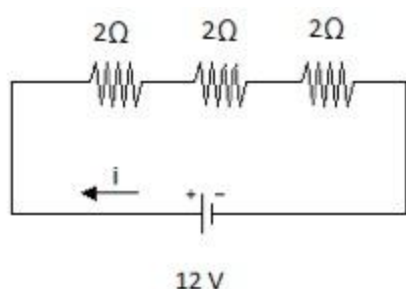
Figura 21: Circuito com apenas resistores e geradores.
