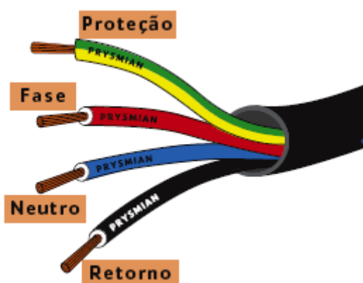
Figura 2: Ilustração dos condutores e suas cores padrão.
