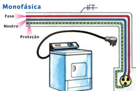
Figura 37: Esquema de ligação de tomadas de uso específico (TUE's - monofásica).
