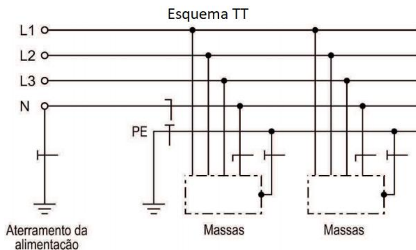
Figura 28: Esquema de aterramento TT.
