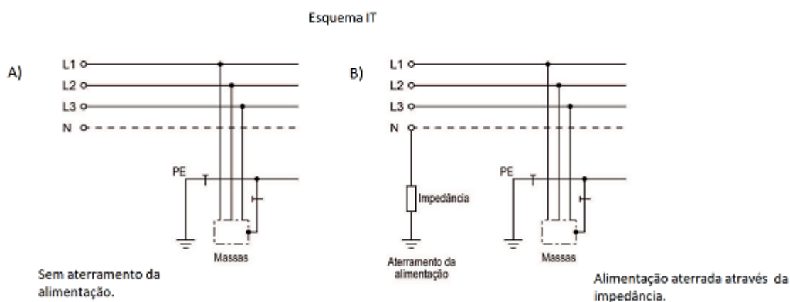
Figura 29: Esquema de aterramento IT.
