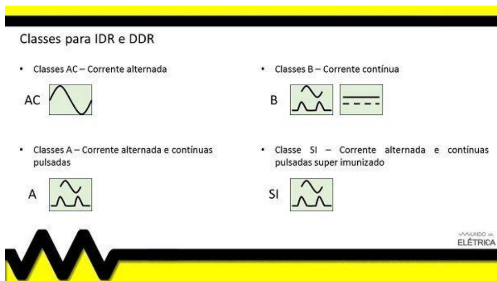
Figura 39: Classes para IDR e DDR.
