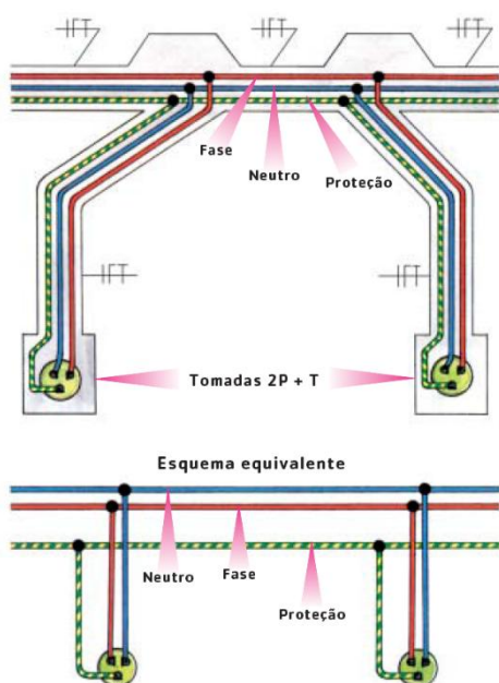
Figura 36: Esquema de ligação de tomadas de uso geral (TUG's).
