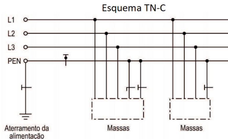
Figura 26: Esquema de aterramento TN-C.
