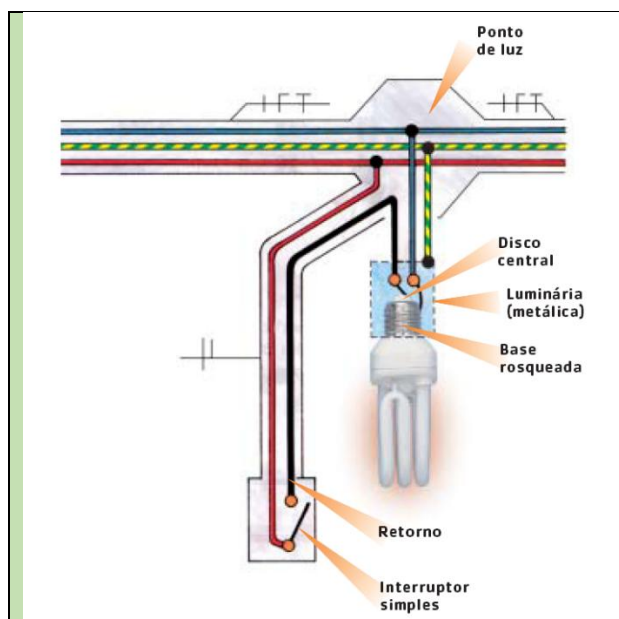
Figura 3: Esquema ilustrativo de um ponto de luz.
