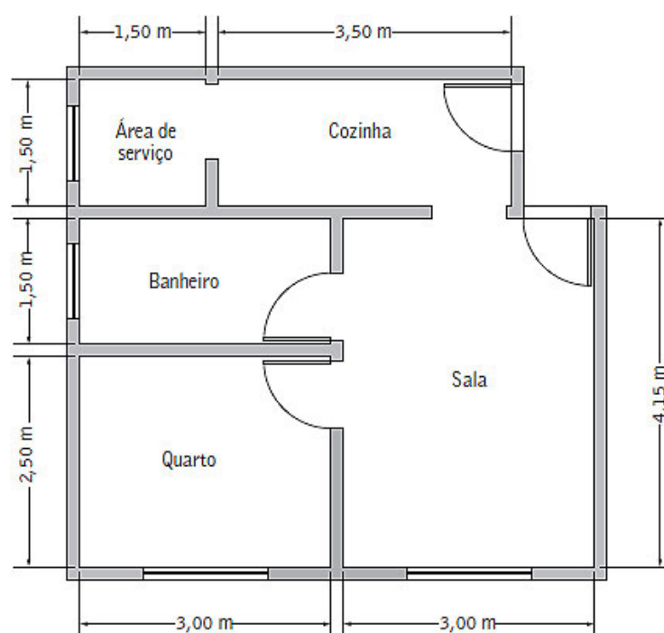
Figura 35: Esboço de uma planta baixa de um apartamento.
