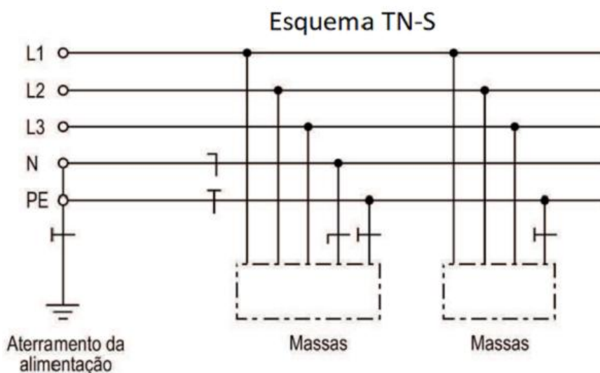
Figura 25: Esquema de aterramento TN-S.
