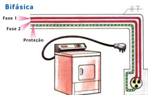
Figura 38: Esquema de ligação de tomadas de uso específico (TUE's - bifásica).
