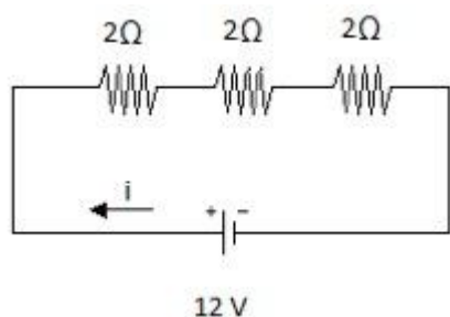
Figura 21: Circuito com apenas resistores e geradores.
