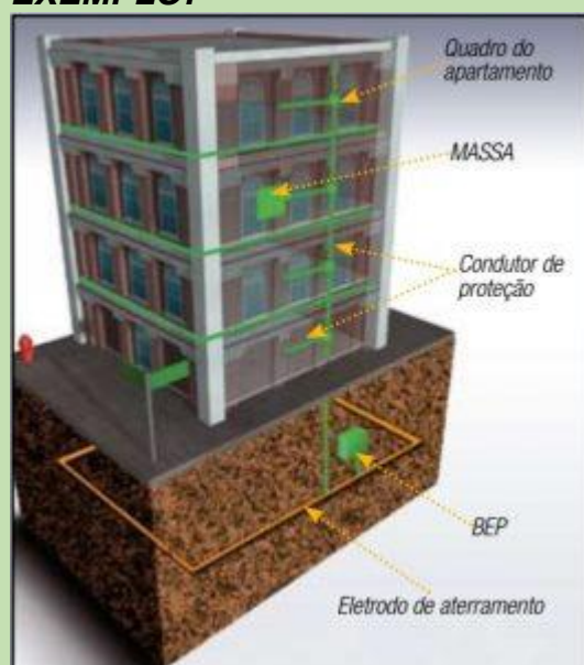
Figura 32: Exemplo de aplicação de um sistema de aterramento e equipotencialização num edifício de apartamentos.
