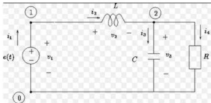
Figura 20: Circuito com indutor (L), capacitor (C), resistor (R), tensão alternada (e(t)).
