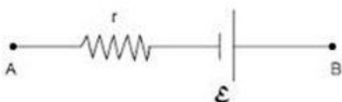
Figura 16: Representação de um gerador no papel.
