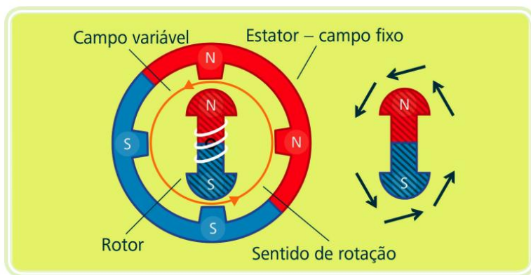
Figura 30: Ação dos campos magnéticos.
