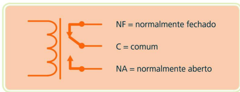
Figura 26: Contatos NF, C e NA com o relé desenergizado.
