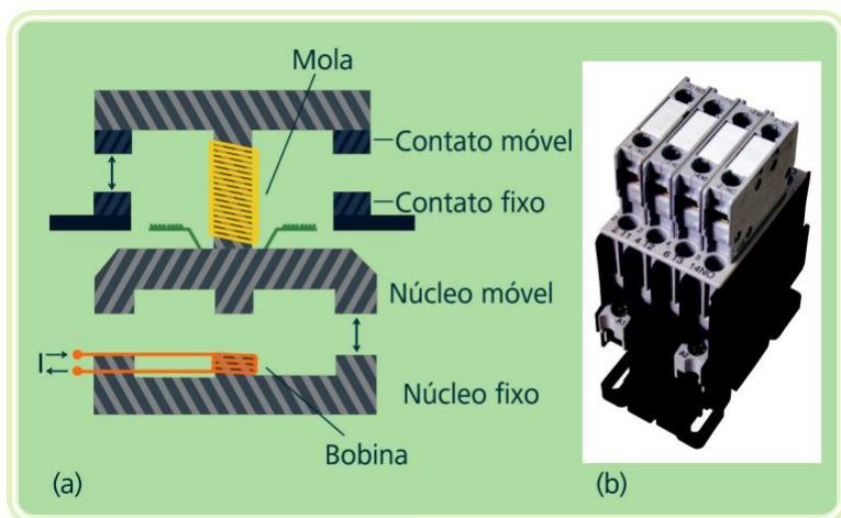
Figura 27: Contator: estrutura simplificada (a) e dispositivo comercial (b).
