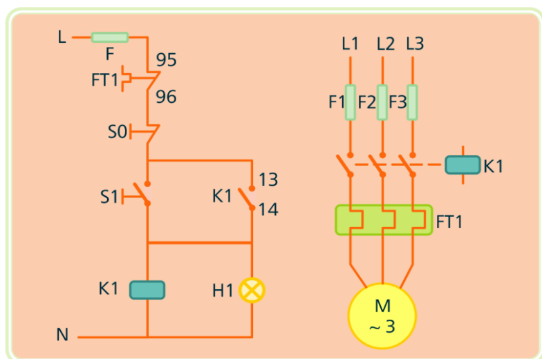
Figura 28: Diagramas de comando e de força de uma partida direta.
