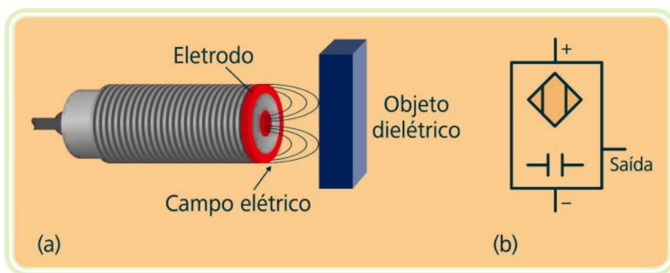
Figura 7: Exemplo de sensor capacitivo.
