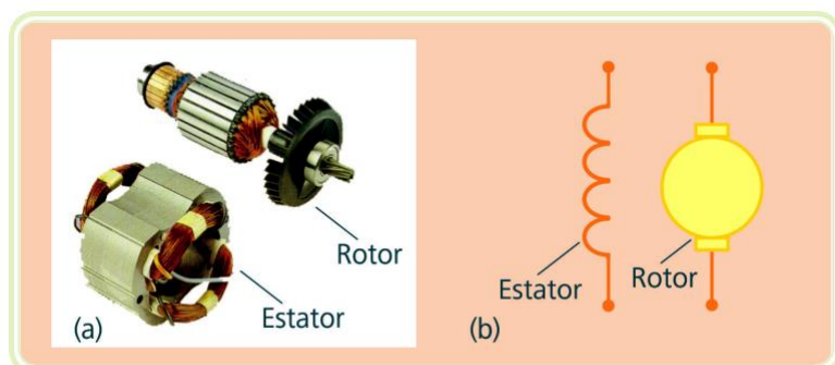
Figura 29: Estator e rotor do motor CC: estruturas (a) e simbologias (b).
