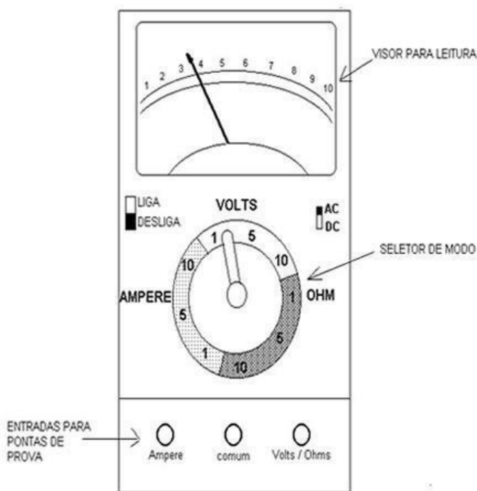
Figura 3: Multímetro.
