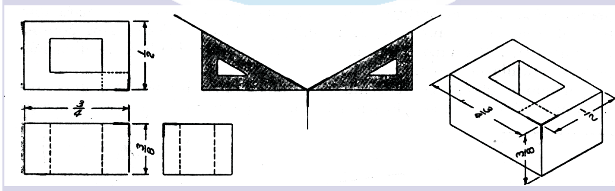
Figura 51 – Eixos isométricos e elaboração da perspectiva
