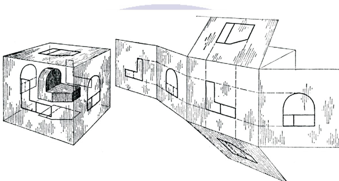
Figura 19 – projeção completa de seis vistas (terceiro diedro) e rebatimento
