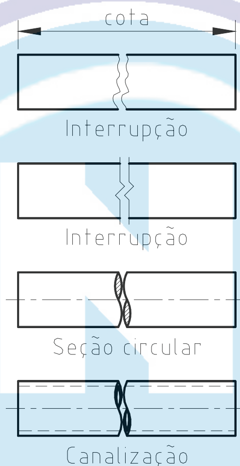
Figura 31 – Exemplo de interrupções
