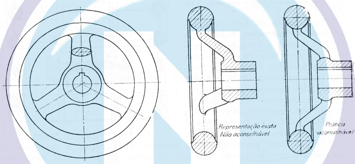
Figura 41 – Representação convencional de um braço de volante
