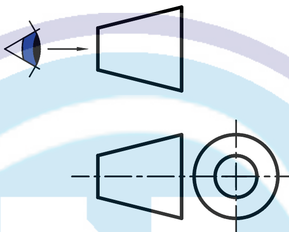
Figura 22 – Denominação de primeiro diedro – ponto de vista e ícone
