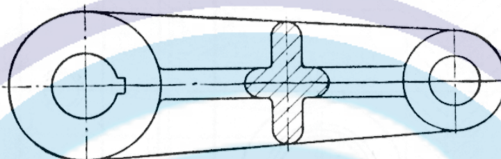
Figura 38 – Exemplo de seção sobre a vista
