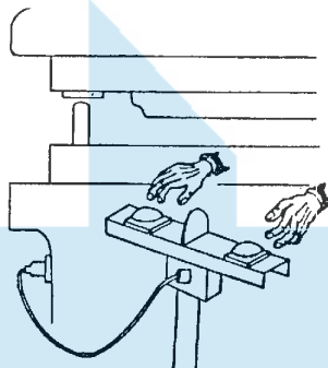
Comando bimanual mantém as mãos ocupadas fora da zona de perigo durante o ciclo da máquina
