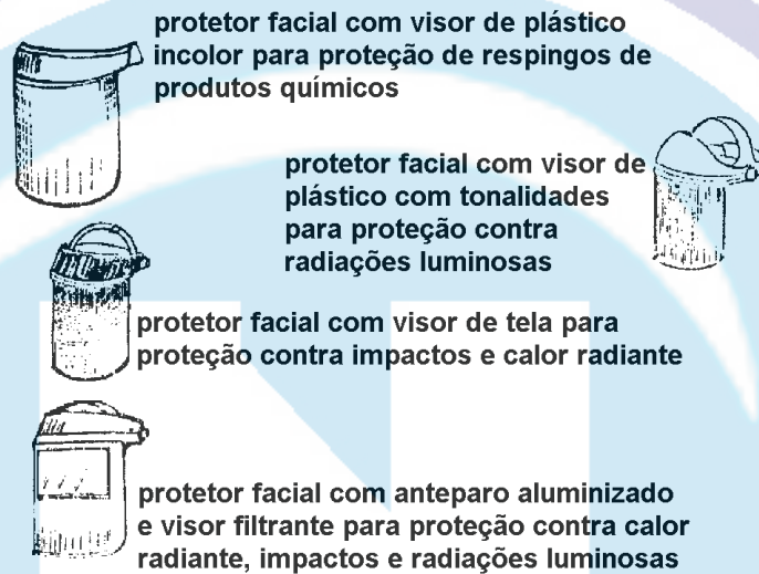
Figura VI.7 – Proteção facial
