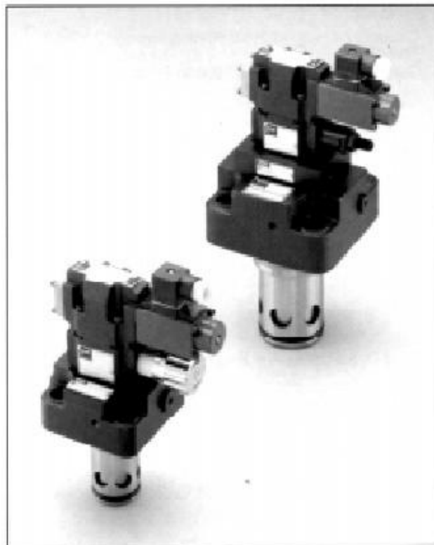
Função de limitadora de alívio de pressão, operada por solenóide proporcional Tamanho nominal 32 e 50
