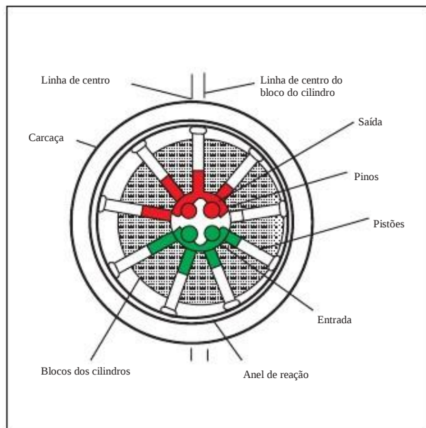
Operação de bomba de pistões radiais
