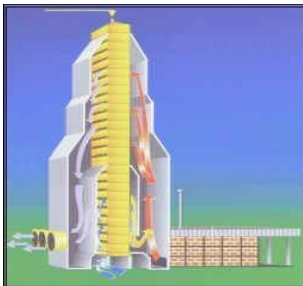
FIGURA - Processo ar quente forçado.
