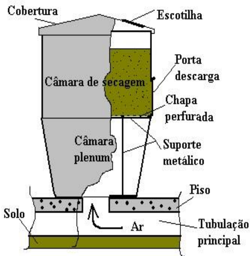
FIGURA - Processo ar forçado sem aquecimento.
