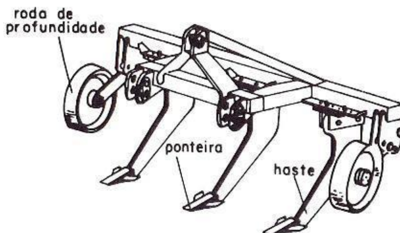
FIGURA - Esquema de um subsolador de 3 hastes.
