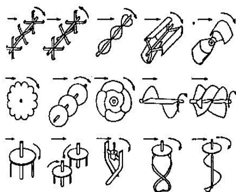
FIGURA - Tipos de Enxadas Rotativas.
