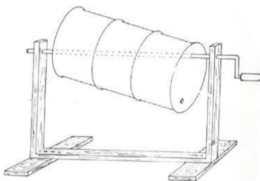
FIGURA -Máquina e tambor giratório para o tratamento de sementes, respectivamente.
