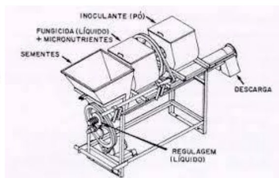
FIGURA -Máquina e tambor giratório para o tratamento de sementes, respectivamente.
