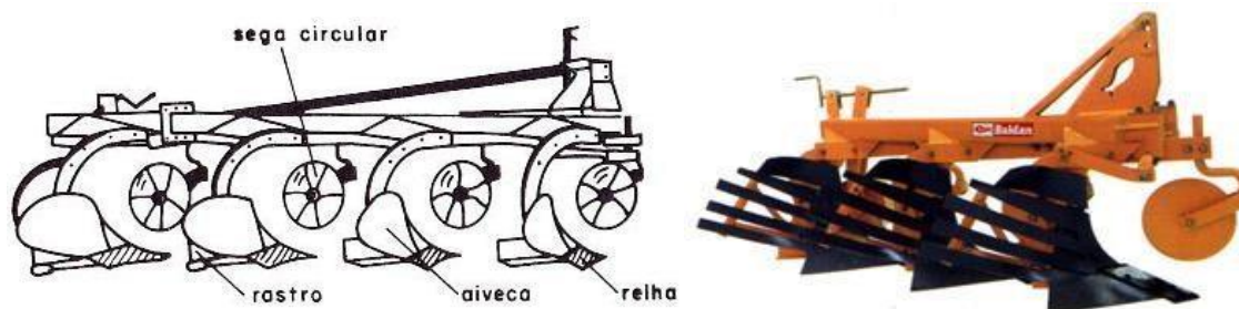
FIGURA - Arado de aivecas.
