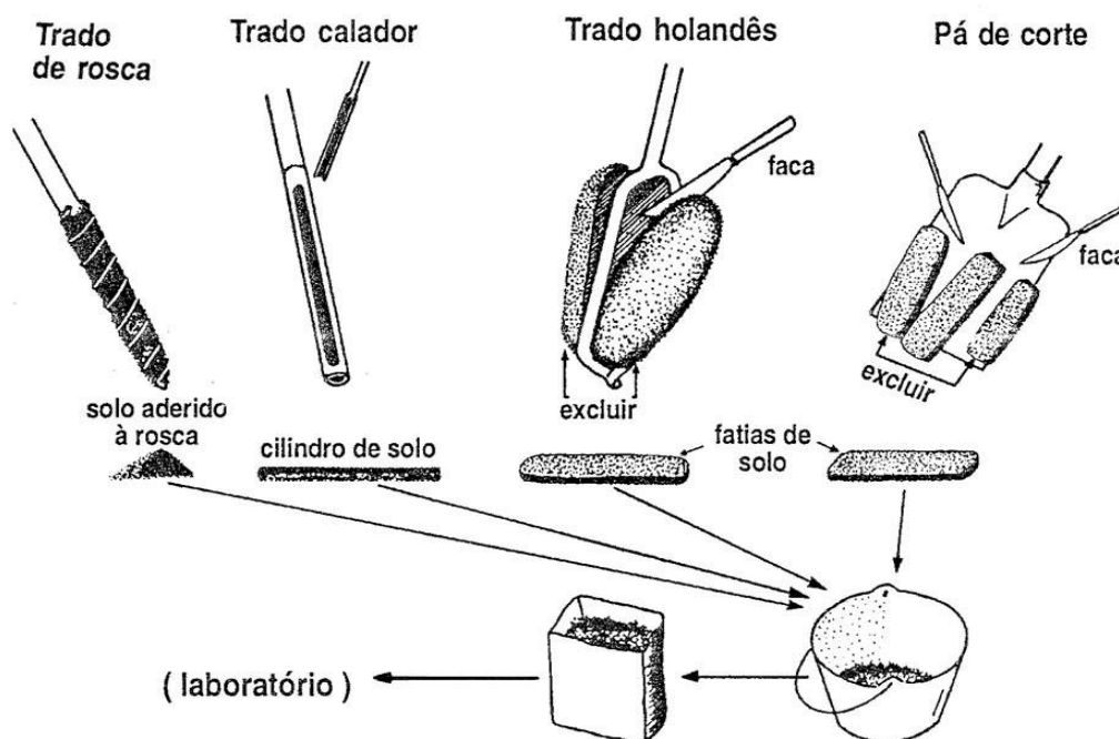
Figura - Equipamentos mais comuns utilizados na coleta de amostras de solo.
