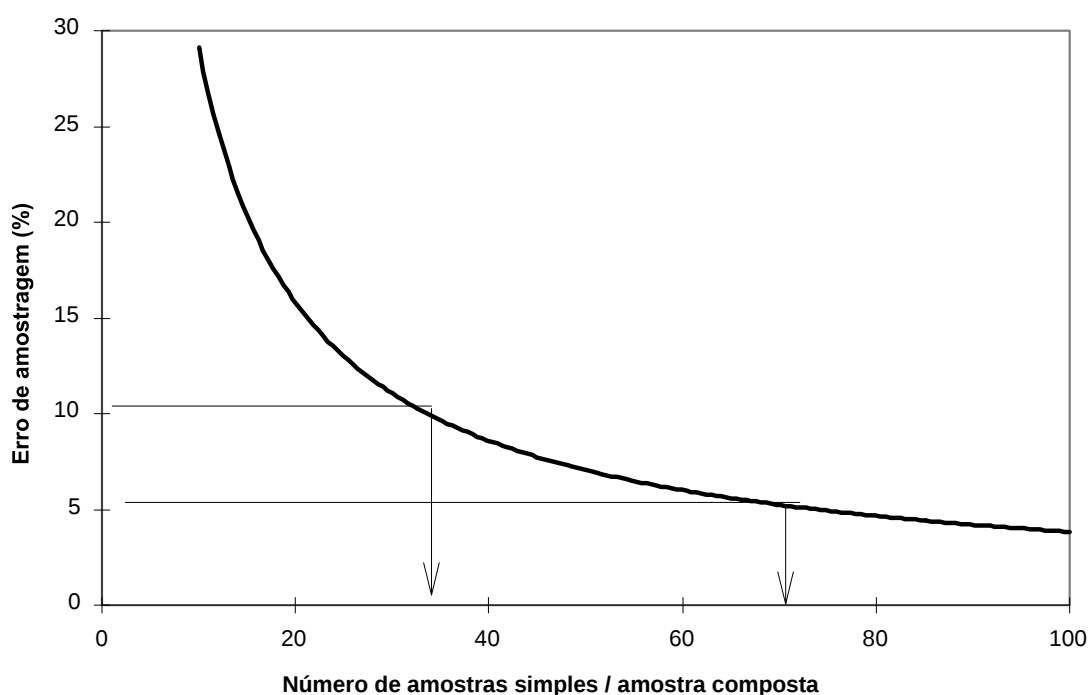
Figura - Variação dos erros de amostragem em função do número de amostras simples por amostra composta.
