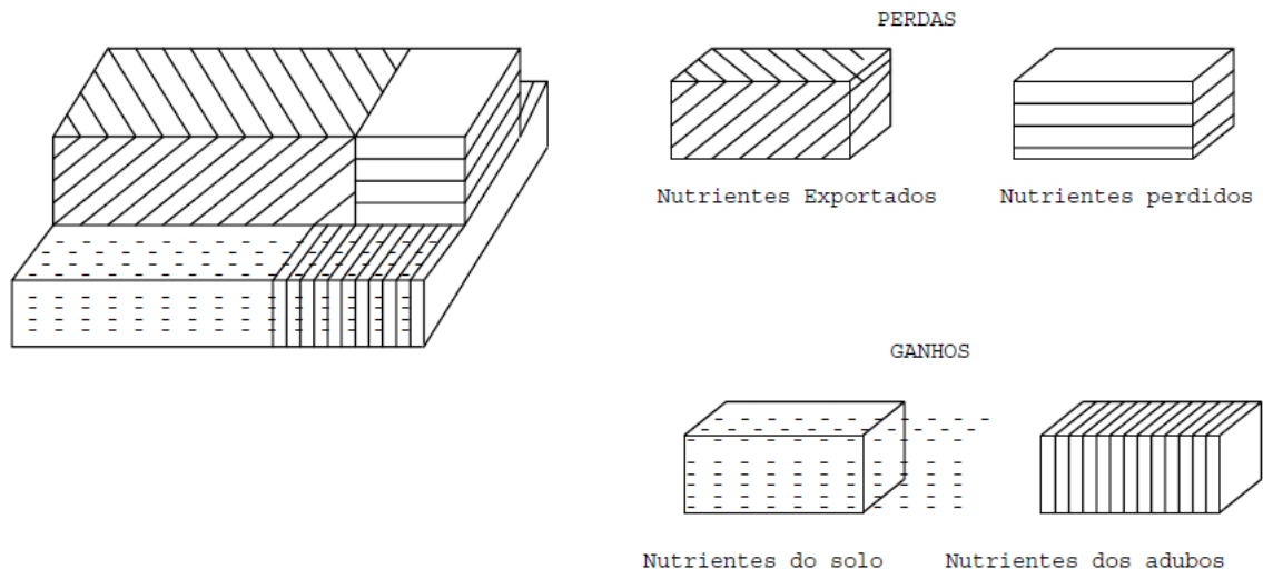
Figura - Representação gráfica da lei da Restituição.
