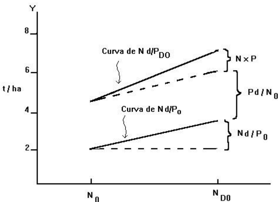
Figura - Efeito do N na ausência de P ( N_d/P_0 ), do P na ausência de N ( P_d/N_0 ) e da interação N, P ( N \times P ).
