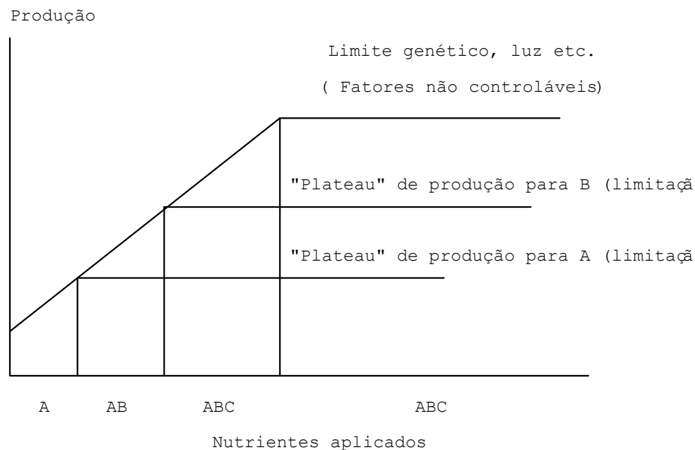
Figura - Resposta linear à adição de nutrientes baseada na Lei do Mínimo.
