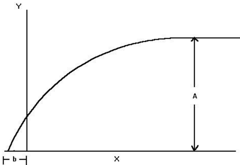
Figura- Representação gráfica da equação de Mitscherlich.
