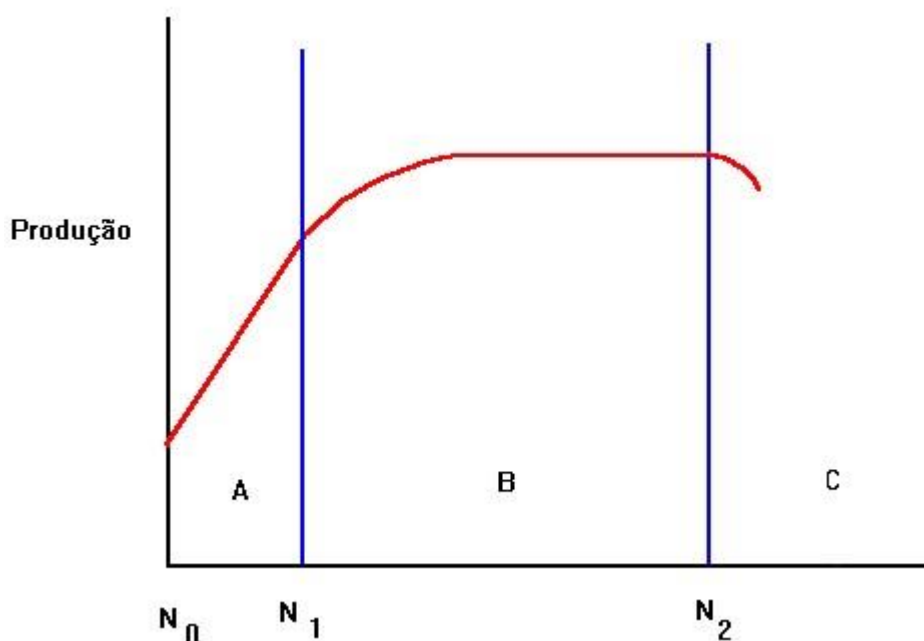
Figura - Curva de resposta à adição de um nutriente.
