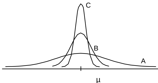
Figura - Distribuições normais com mesma média e desvios padrão diferentes
