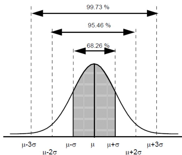
Figura - Probabilidades da distribuição normal
