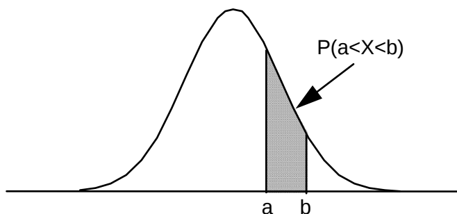
Figura – Probabilidade como área sob a curva entre dois pontos
