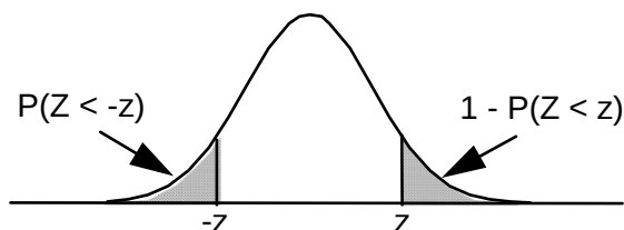
Figura - Áreas correspondentes na distribuição normal
