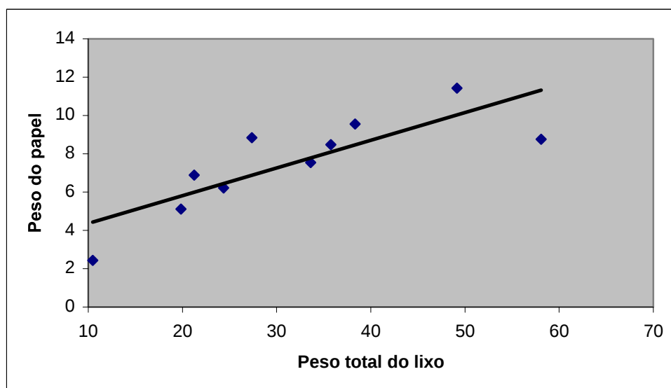
Figura - Correlação entre o peso total do lixo descartado e o peso do papel contido nesse lixo
