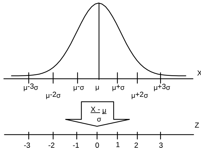
Figura - Transformação de uma N(\mu, \sigma^2) para uma N(0,1)
