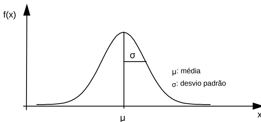
Figura - Curva normal típica
